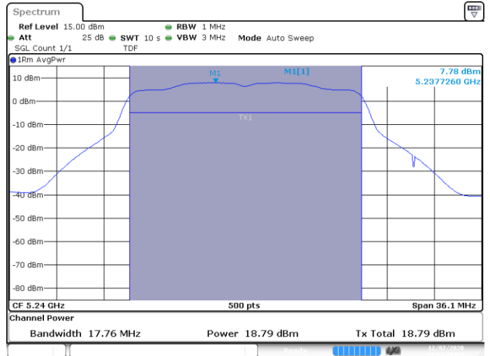
MIMO B-802.11n-20MHz-Ch48-5240MHz-HT8
