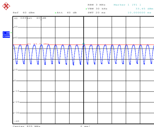
835MHz - CW
