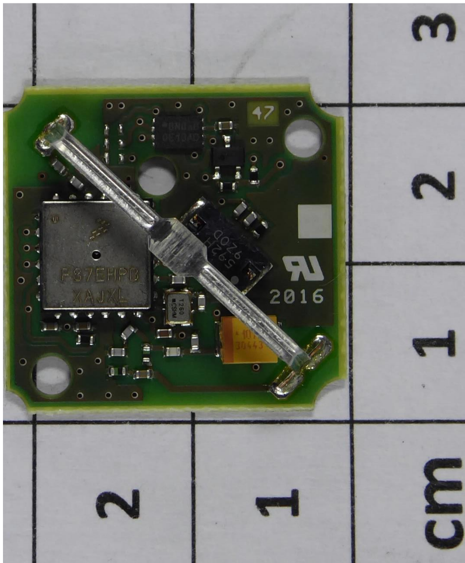
PCB top
