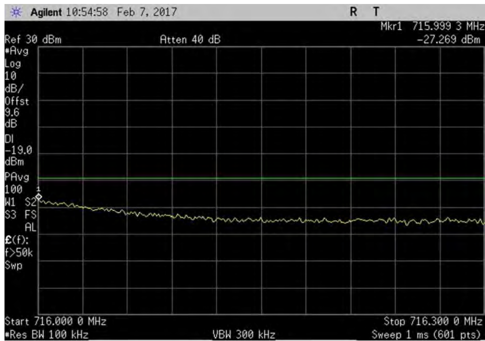
7.5_OBE_UL_698-716MHz_H_PreAGC_LTE
