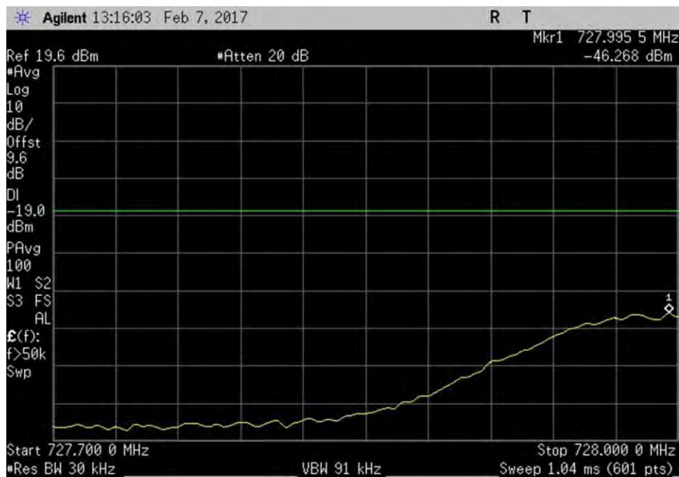
7.5_OBE_DL_728-746MHz_L_PreAGC_GSM
