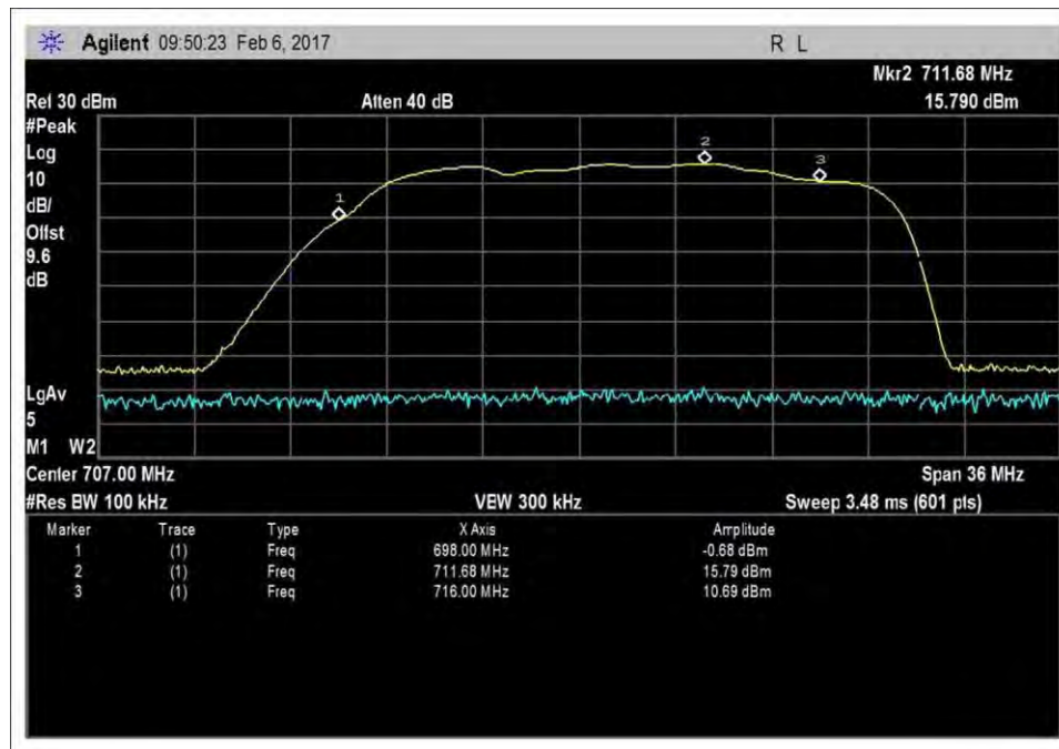
7.1_Band Verify_UL_698-716MHz
