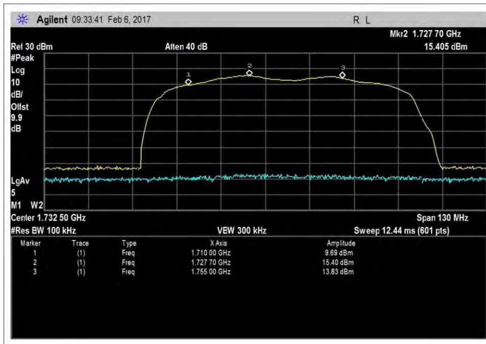
7.1_Band Verify_UL_1710-1755MHz_Zoom
