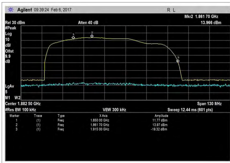
7.1_Band Verify_UL_1850-1915MHz
