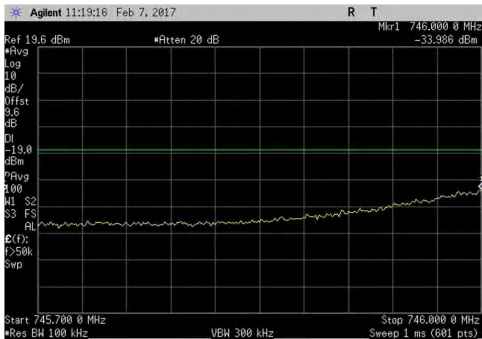
7.5_OBE_DL_746-757MHz_L_PreAGC_LTE
