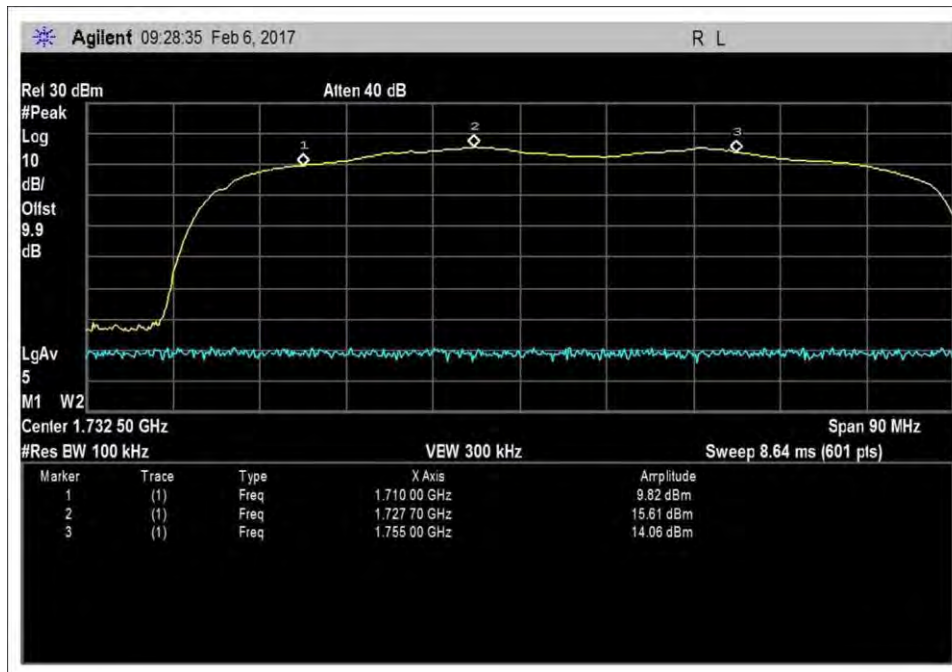
7.1_Band Verify_UL_1710-1755MHz
