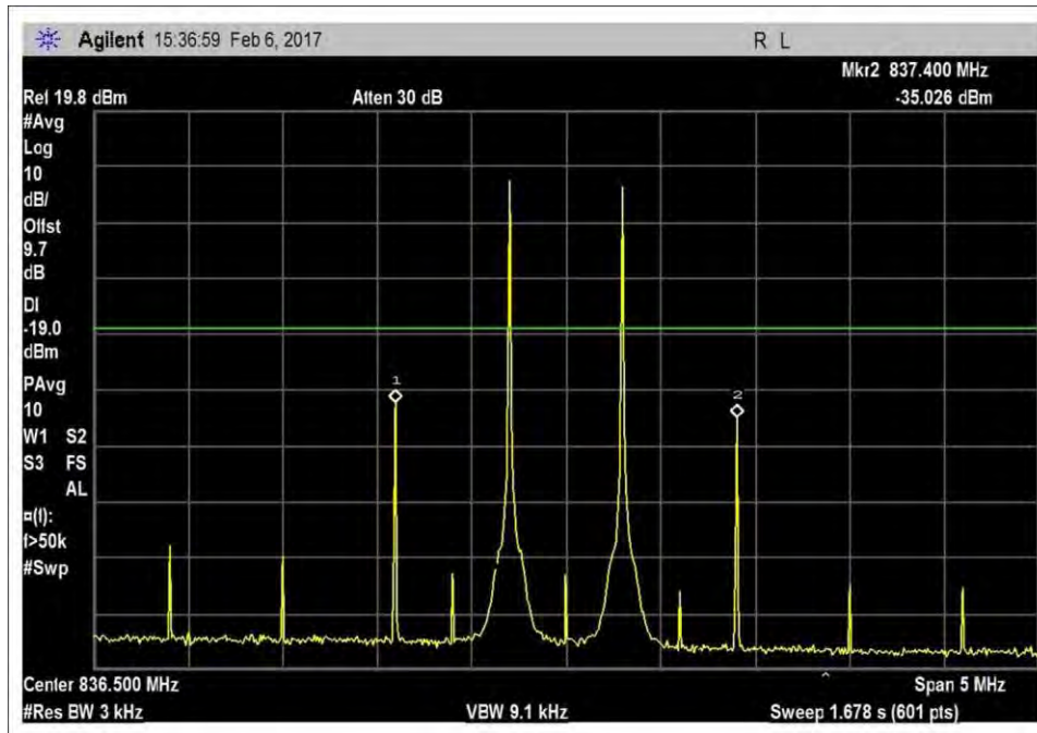
7.4_Intermod_UL_824-849MHz
