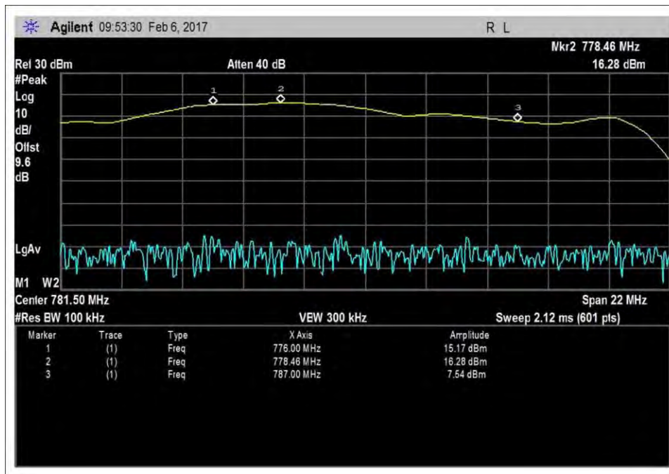
7.1_Band Verify_UL_776-787MHz
