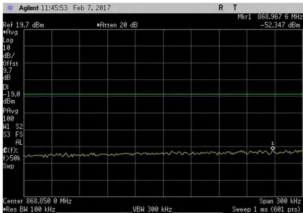
7.5_OBE_DL_869-894MHz_L_PreAGC_CDMA
