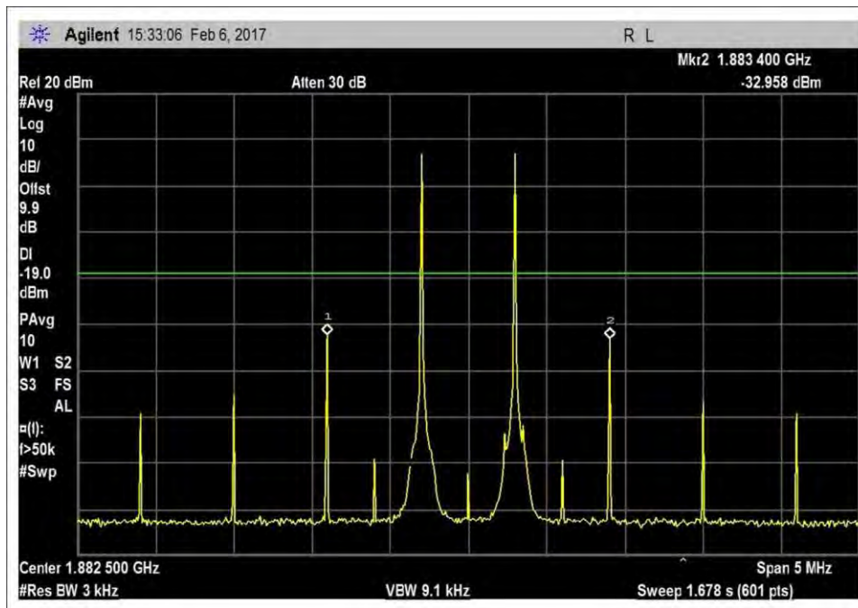
7.4_Intermod_UL_1850-1915MHz
