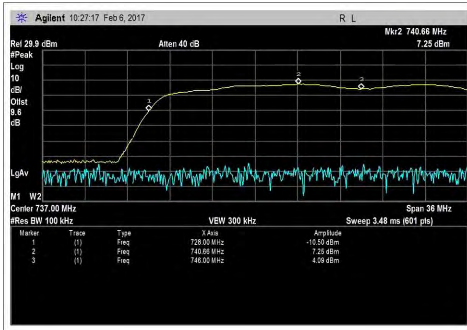
7.1_Band Verify_DL_728-746MHz
