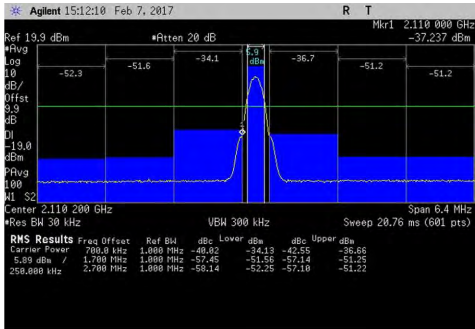
7.5_OBE_DL_2110-2155MHz_L_PreAGC_GSM
