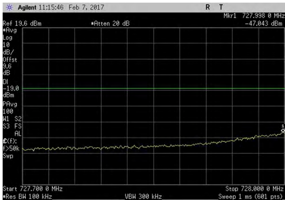
7.5_OBE_DL_728-746MHz_L_PreAGC_LTE
