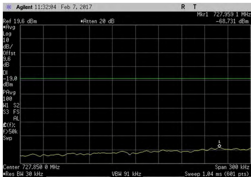
7.5_OBE_DL_728-746MHz_L_PreAGC_CDMA.
