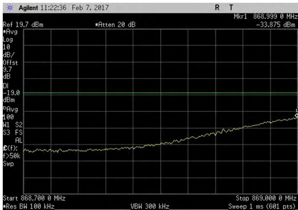
7.5_OBE_DL_869-894MHz_L_PreAGC_LTE
