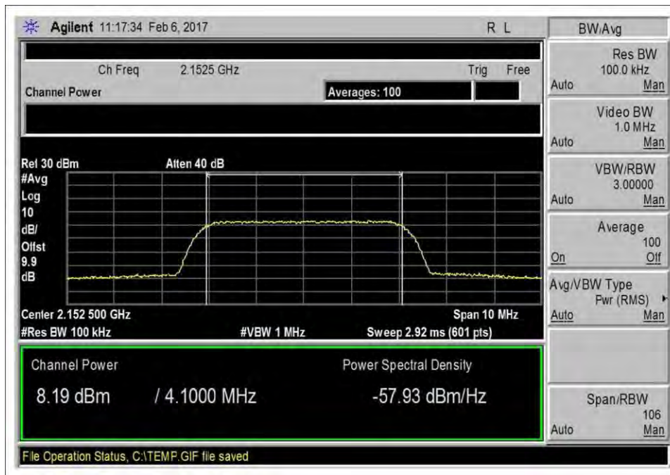
7.2_Power_DL_2110-2155MHz
