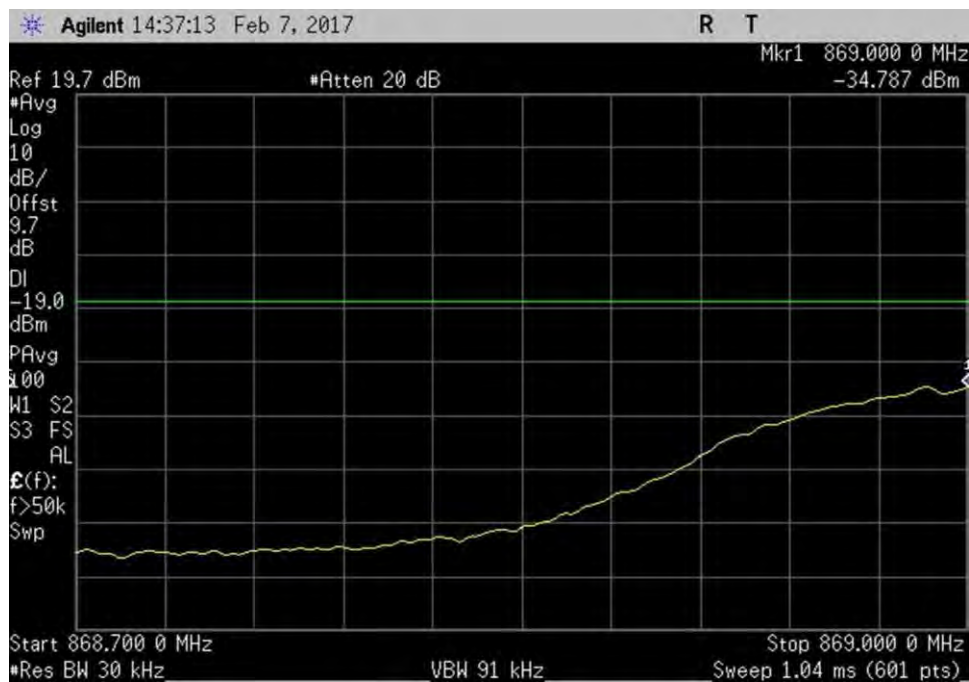
7.5_OBE_DL_869-894MHz_L_PreAGC_GSM
