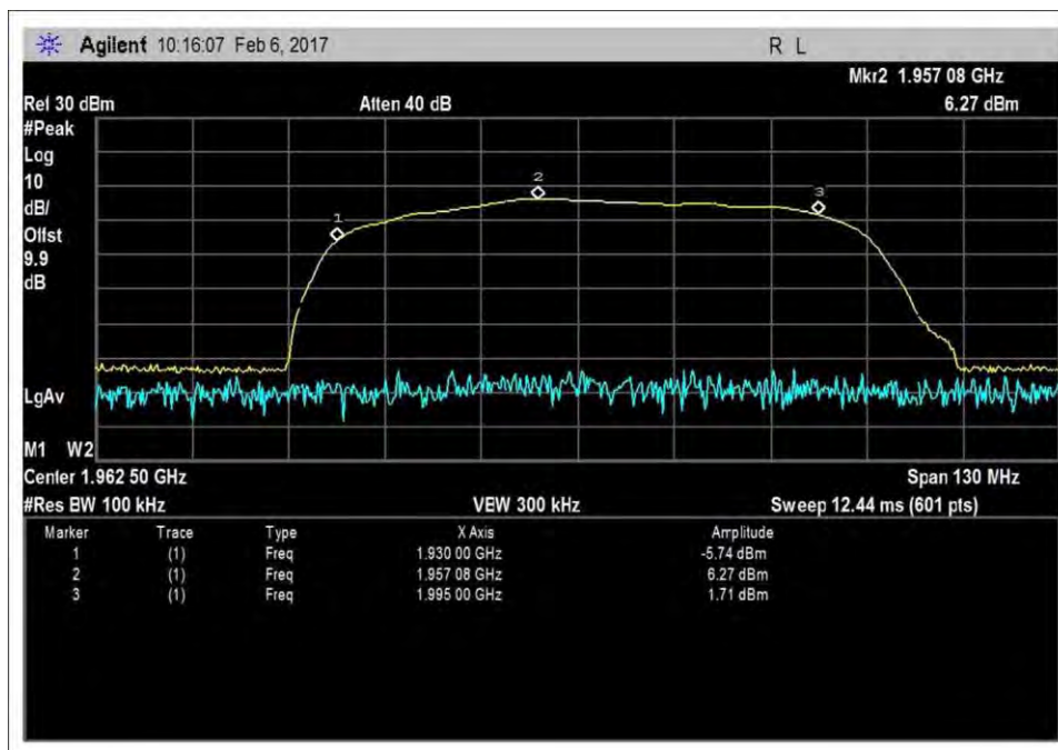
7.1_Band Verify_DL_1930-1995MHz
