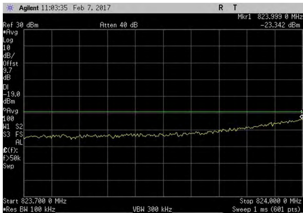
7.5_OBE_UL_824-849MHz_L_PreAGC_LTE.
