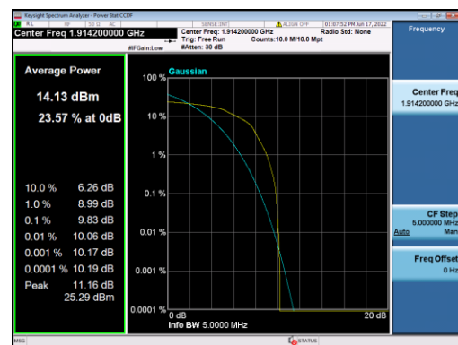
B25-5M-Low CH-PAPR-Q16
