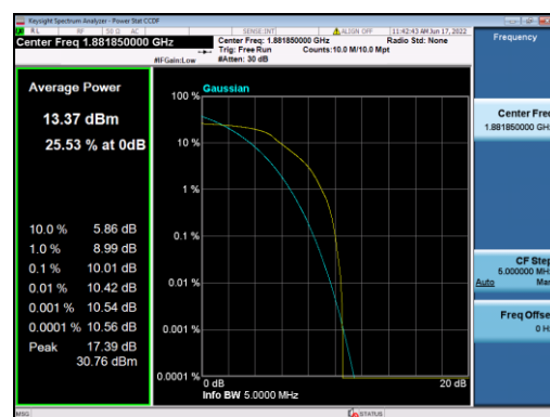
B25-3M-Mid CH-PAPR-QPSK
