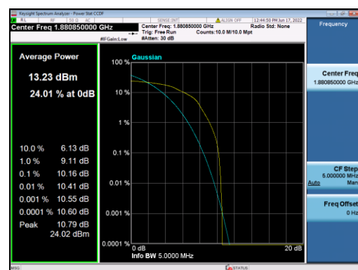
B25-5M-Mid CH-PAPR-Q16
