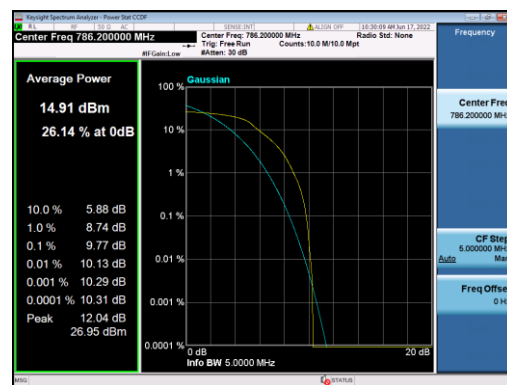
B13-5M-Low CH-PAPR-QPSK
