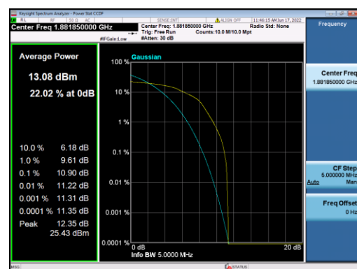
B25-3M-Mid CH-PAPR-Q16
