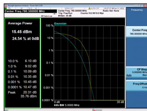
B13-5M-Mid CH-PAPR-Q16
