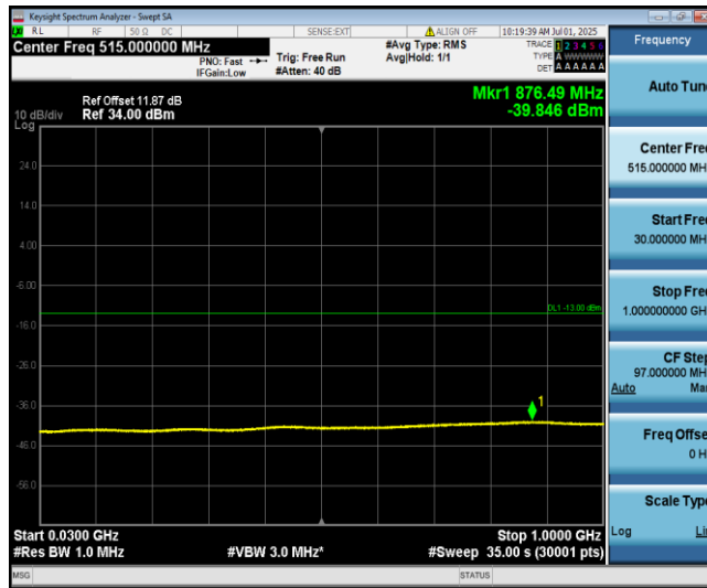
Band4-1.4MHz-QPSK-20175-1-0-Low-30-1000--39.85-PASS
