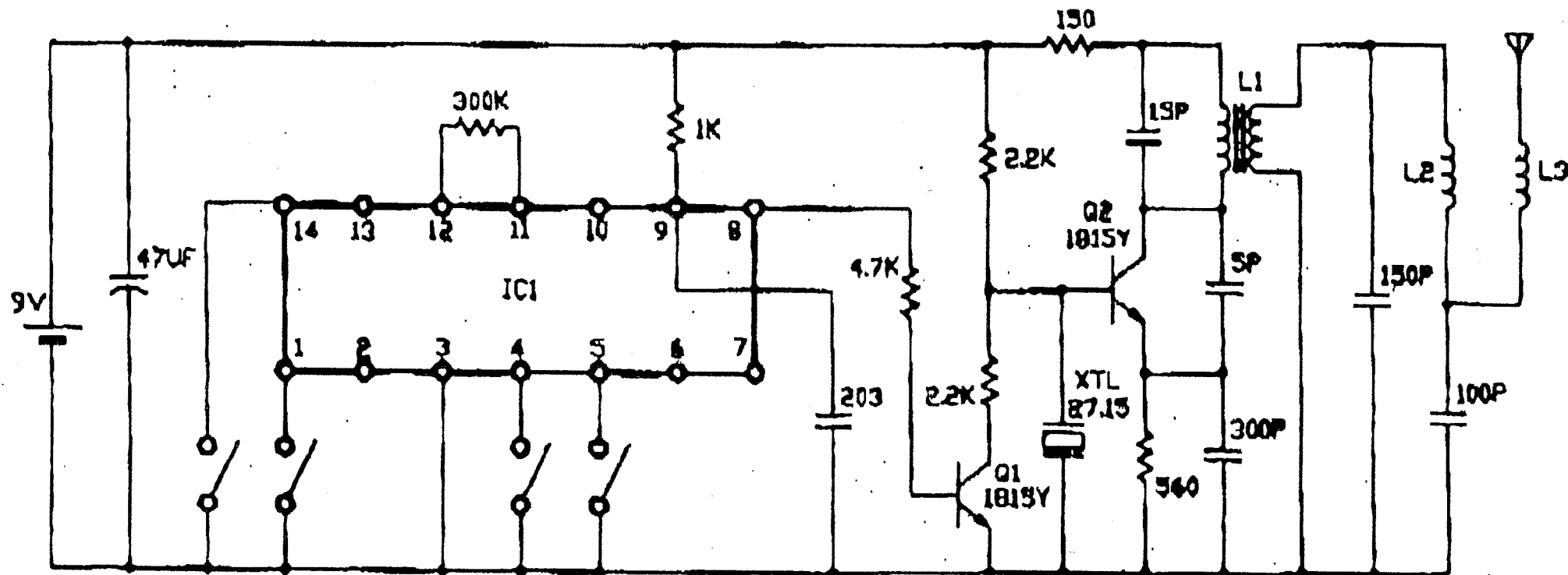
现电路
