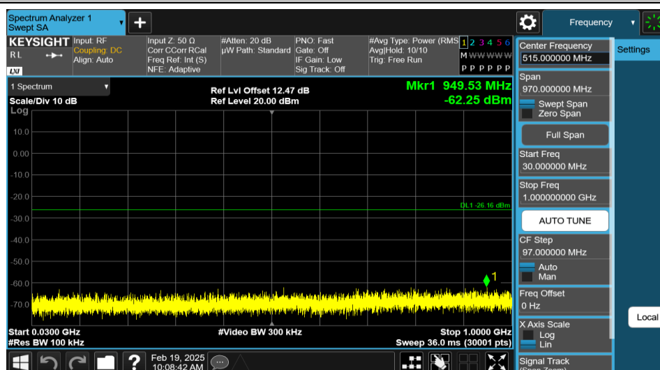
11G-Ant1-2412-30~1000-PASS
