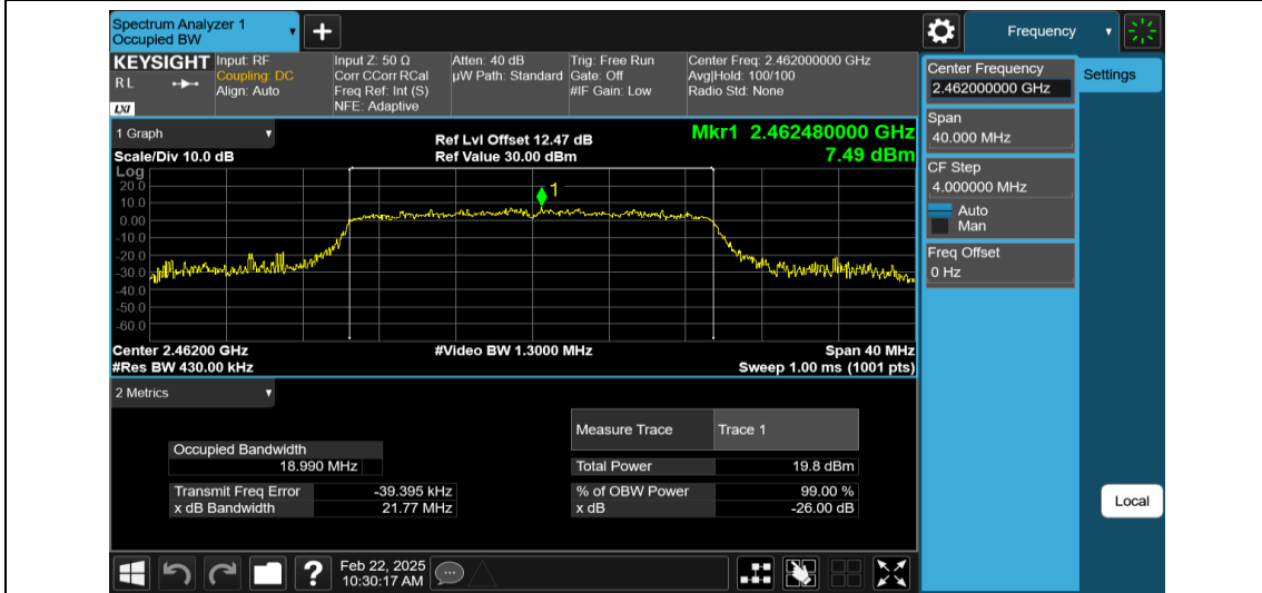
11AX20MIMO-Ant1-2462
