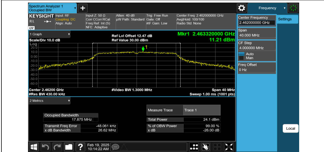
11G-Ant1-2462
