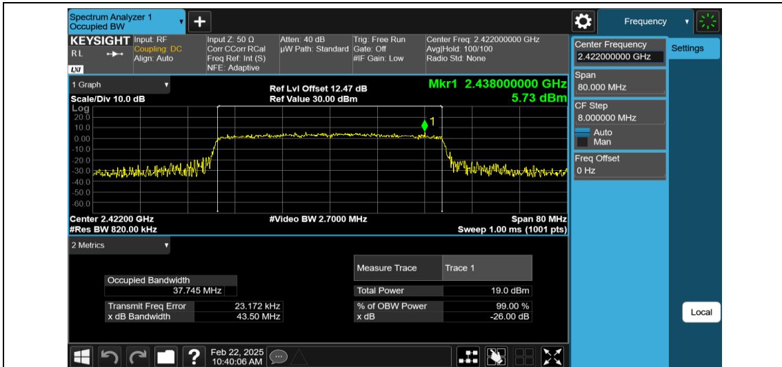
11AX40MIMO-Ant1-2422
