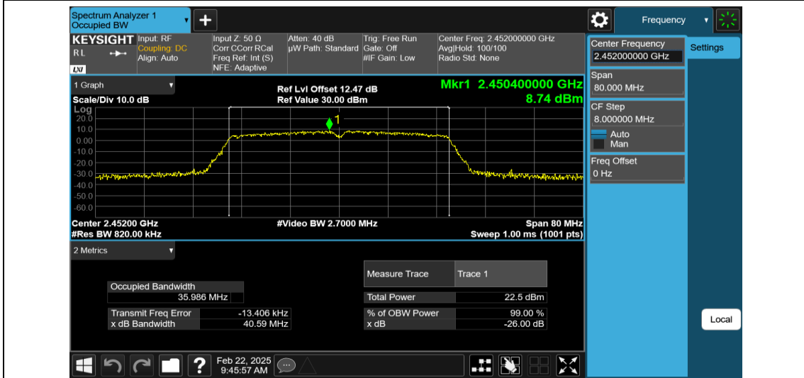
11N40MIMO-Ant1-2452
