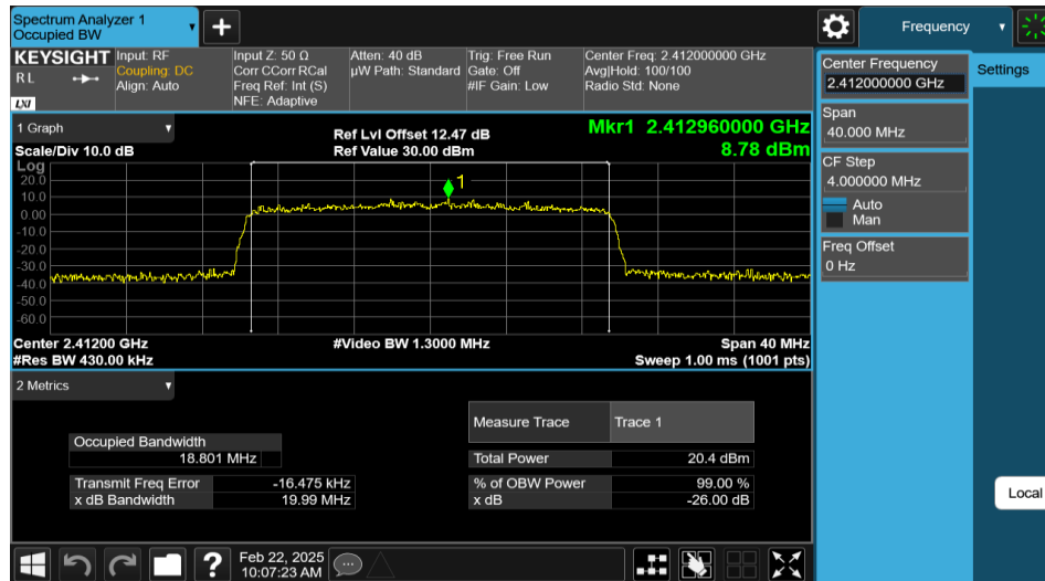
11AX20MIMO-Ant1-2412
