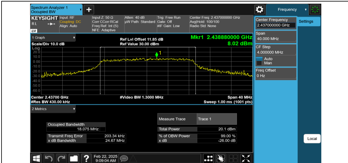
11N20MIMO-Ant2-2437
