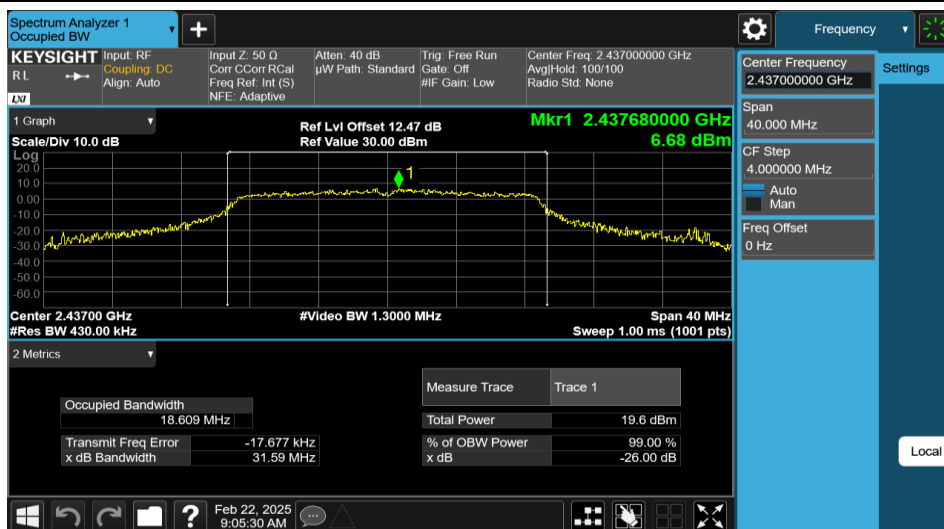
11N20MIMO-Ant1-2437
