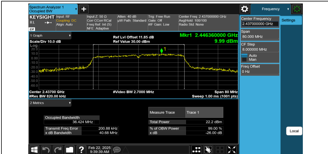
11N40MIMO-Ant2-2437
