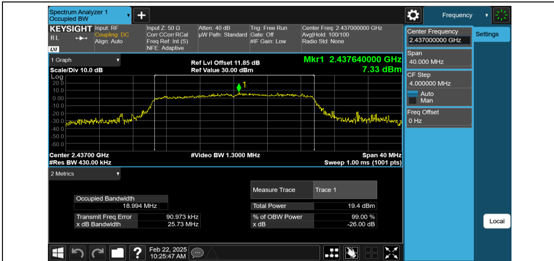
11AX20MIMO-Ant2-2437
