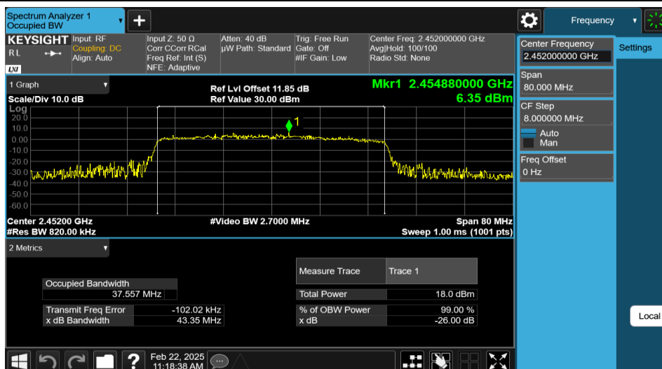
11AX40MIMO-Ant2-2452
