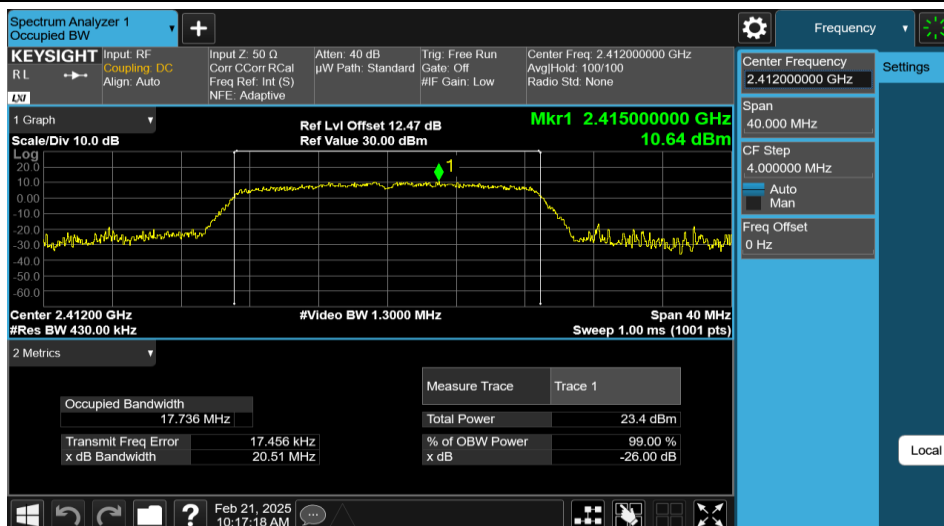
11N20MIMO-Ant1-2412
