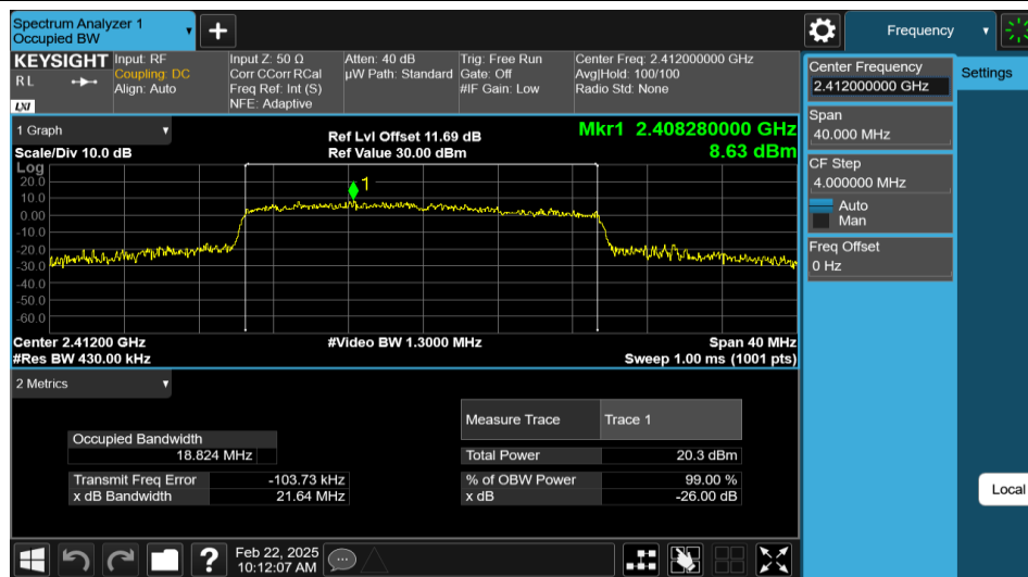
11AX20MIMO-Ant2-2412
