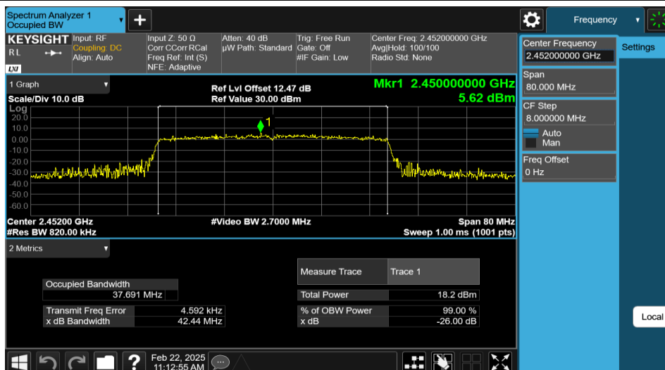
11AX40MIMO-Ant1-2452
