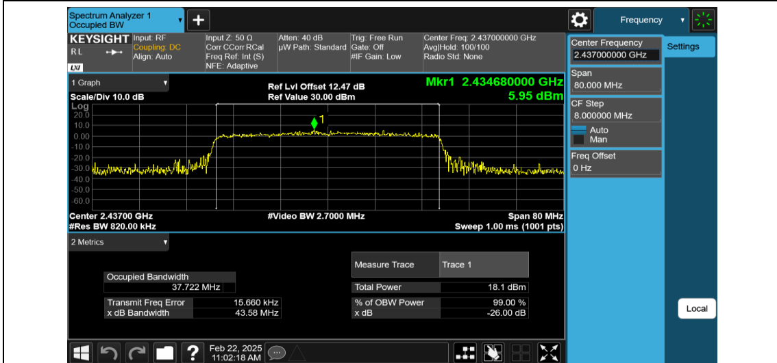
11AX40MIMO-Ant1-2437
