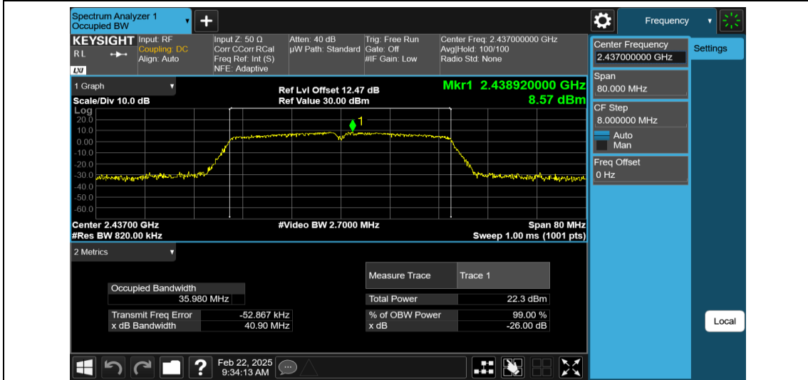
11N40MIMO-Ant1-2437
