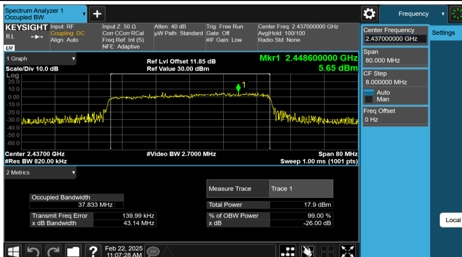
11AX40MIMO-Ant2-2437
