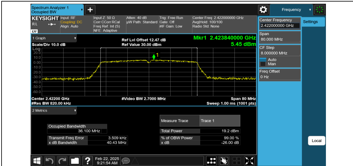
11N40MIMO-Ant1-2422
