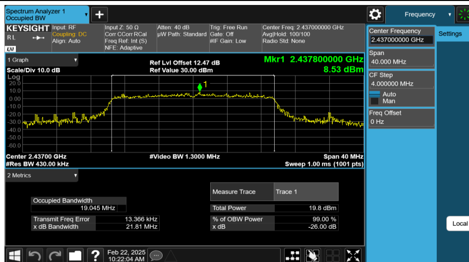
11AX20MIMO-Ant1-2437
