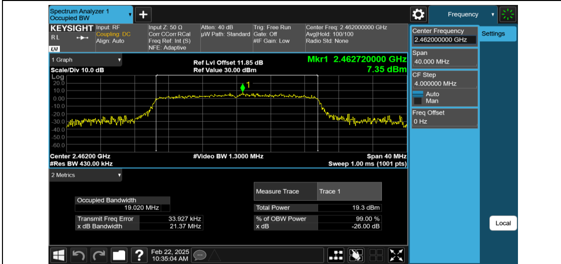
11AX20MIMO-Ant2-2462
