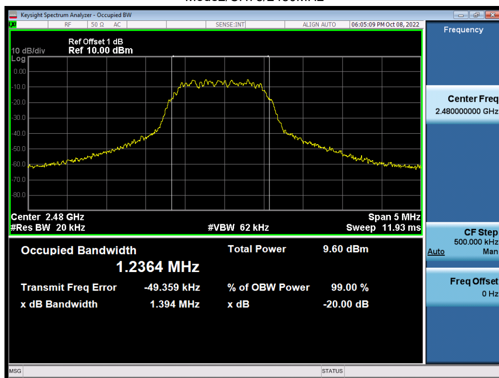
Mode2/CH78/2480MHz
