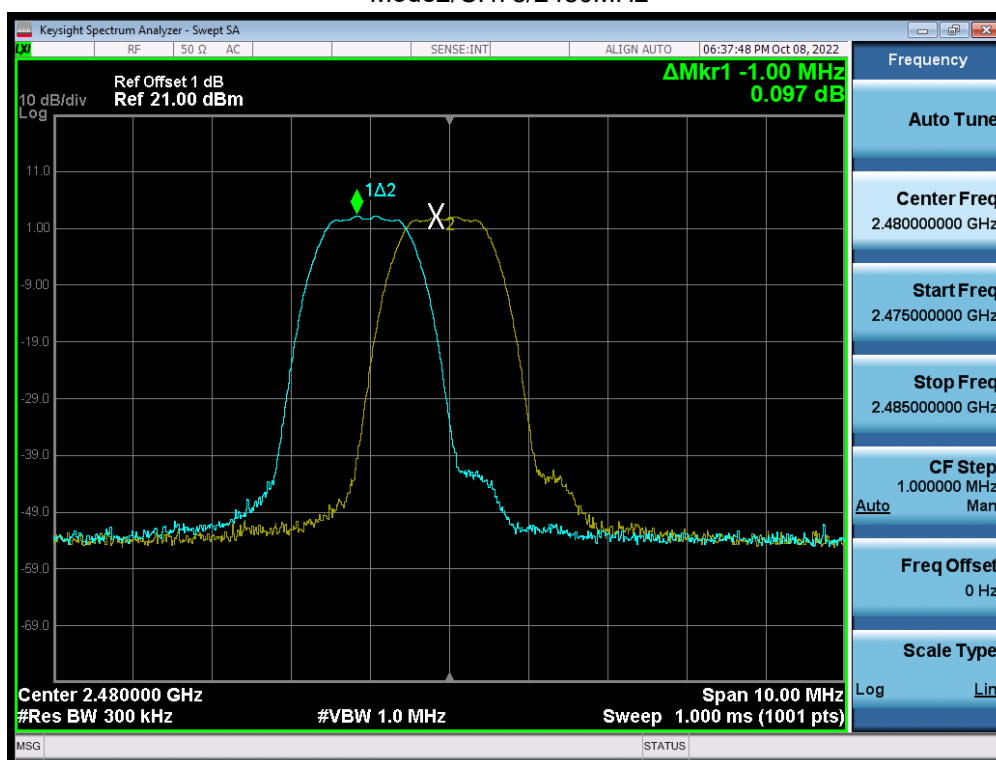
Mode2/CH78/2480MHz
