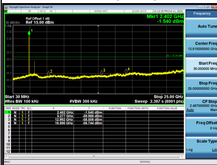
Mode 2 CH00(2402MHz)
