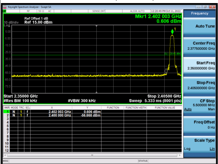
Mode 2 CH00(2402MHz)
