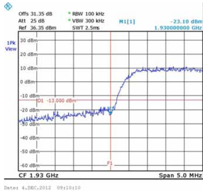
Figure 246.— 1932.50 MHz
