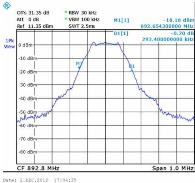
Figure 44.— Input 892.8 MHz.
