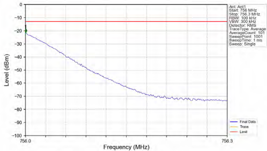
Band13_755.8MHz_GMSK_SISO_Ant1_NTNV_AGC
