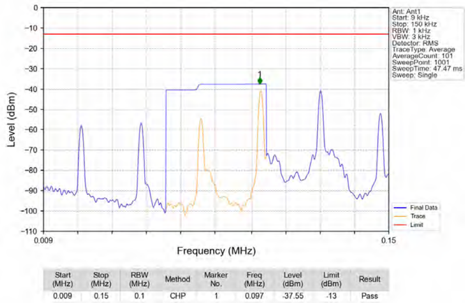
Band13_751MHz_GMSK_SISO_Ant1_NTNV
