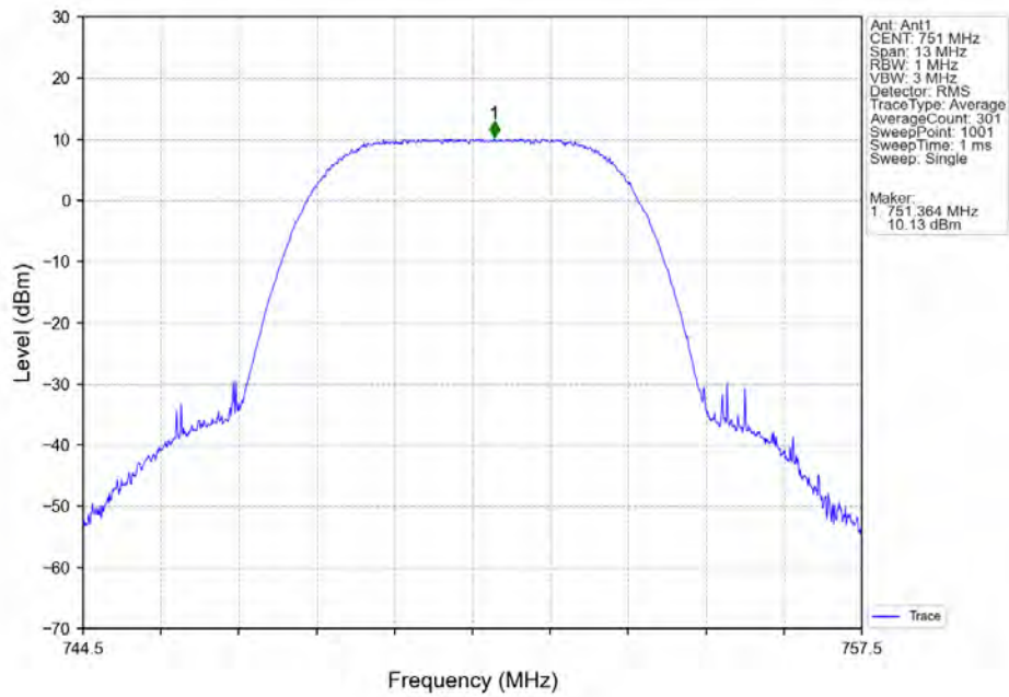
Band13_751MHz_AWGN_SISO_Ant1_NTNV_AGC+3
