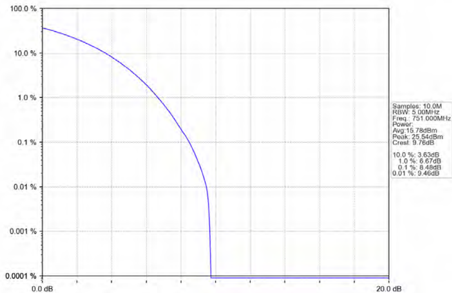
Band13_751MHz_AWGN_SISO_Ant1_NTNV_AGC+3
