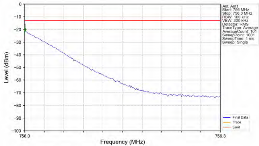
Band13_755.8MHz_GMSK_SISO_Ant1_NTNV_AGC+3
