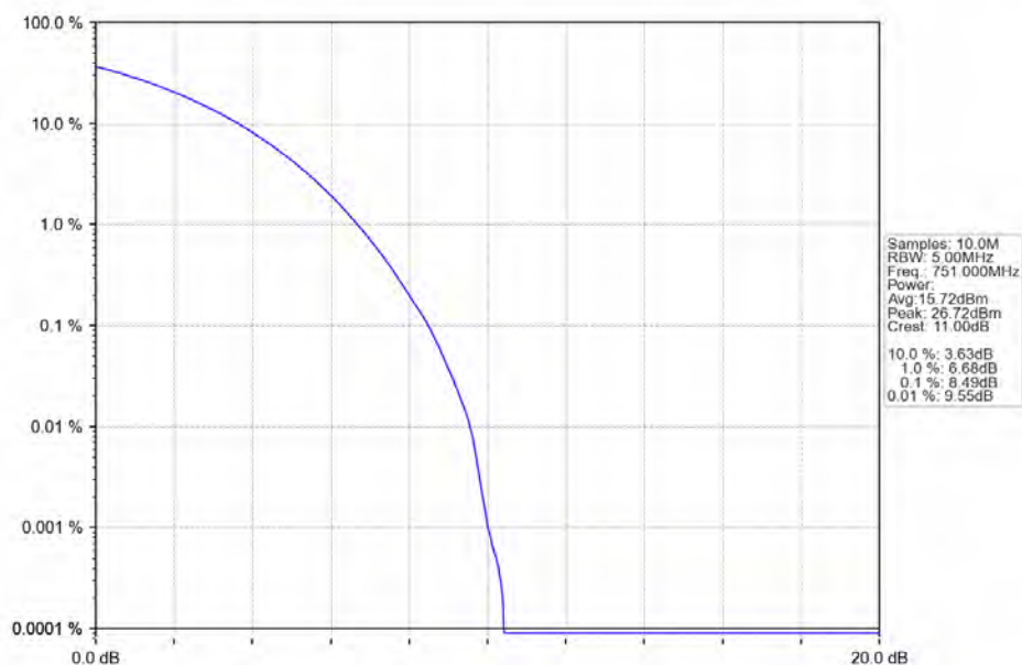
Band13_751MHz_AWGN_SISO_Ant1_NTNV_AGC
