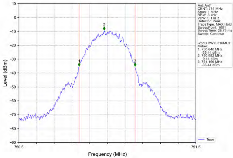
Band13_751MHz_GMSK_SISO_Ant1_NTNV_Input_AGC+3
