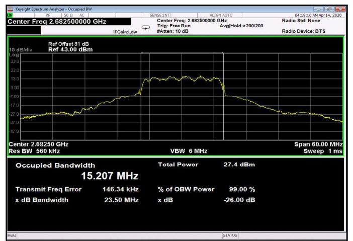
Figure 318: 16QAM 15MHz B.W.; 2682.5MHz, 15kHz Output
