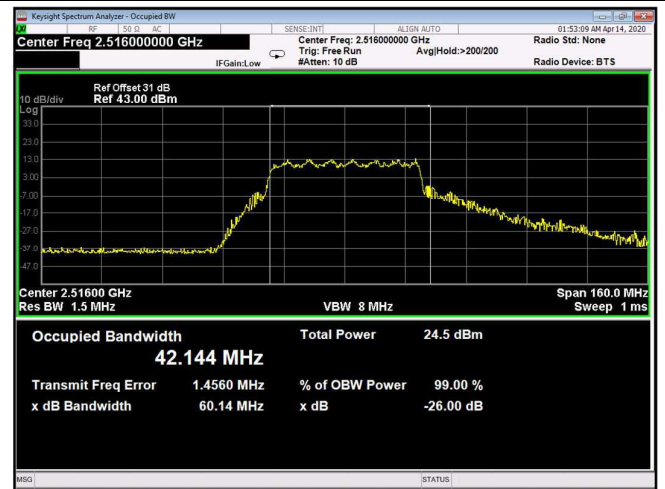
Figure 330: 16QAM 40MHz B.W.; 2516.0MHz, 15kHz Output
