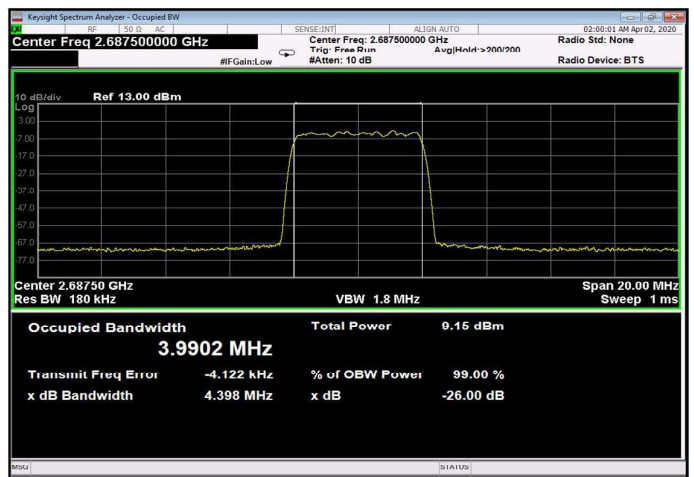
Figure 158: 16QAM 5MHz B.W.; 2687.5MHz, 30kHz Input
