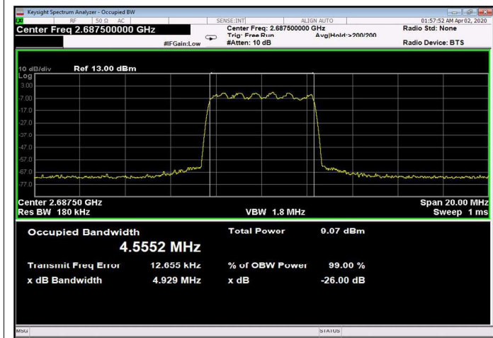
Figure 157: 16QAM 5MHz B.W.; 2687.5MHz, 15kHz Input
