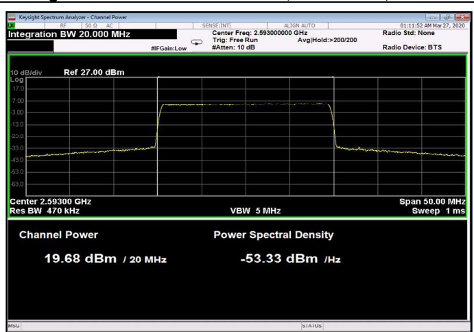
Figure 84: 64QAM 20MHz B.W.; 2593.0MHz, 15kHz
