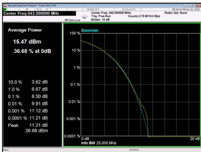
Figure 253: 16QAM 20MHz B.W; 642.0MHz, 15kHz
