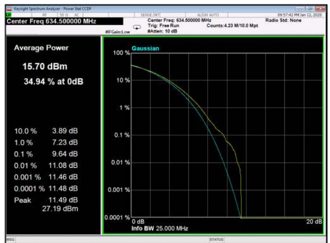
Figure 357: QPSK 20MHz B.W; 634.5MHz, 60kHz
