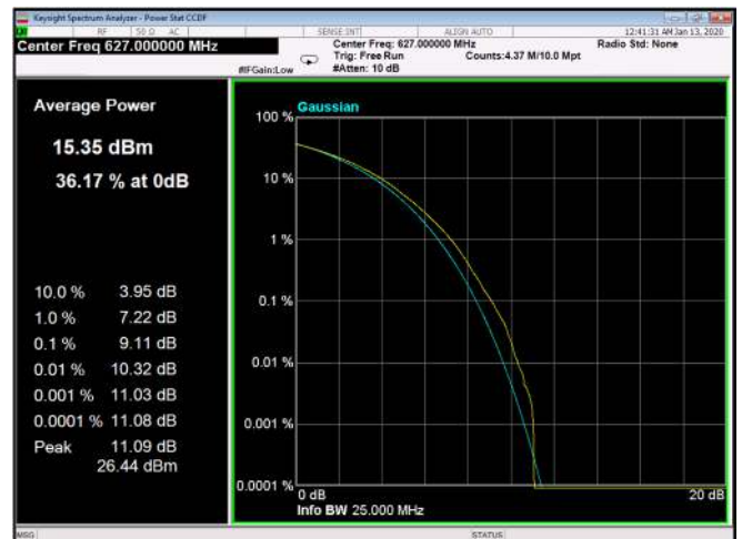
Figure 285: 64QAM 20MHz B.W; 627.0MHz, 30kHz
