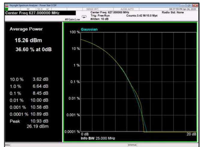
Figure 254: 16QAM 20MHz B.W; 627.0MHz, 30kHz
