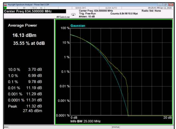
Figure 339: QPSK 10MHz B.W; 634.5MHz, 60kHz
