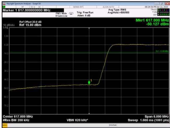
Figure 201: 256QAM 20MHz B.W.; 617.0MHz, 30kHz Lower Edge
