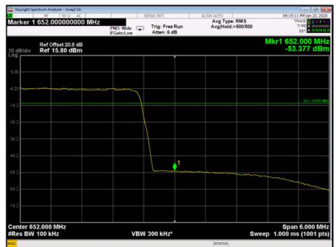
Figure 168: 64QAM 10MHz B.W.; 652.0MHz, 30kHz Upper Edge
