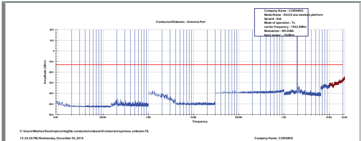
Figure 135 WCDMA - 1932.5 MHz
