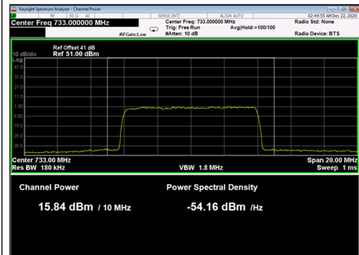
Figure 50: 64QAM 10MHz B.W.; 733.0MHz, 60kHz
