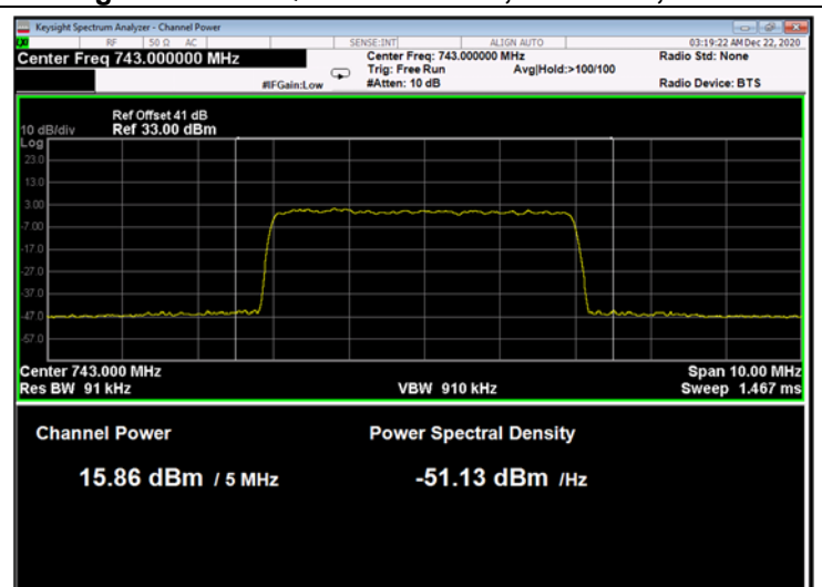
Figure 78: 256QAM 5MHz B.W.; 743.0MHz, 30kHz
