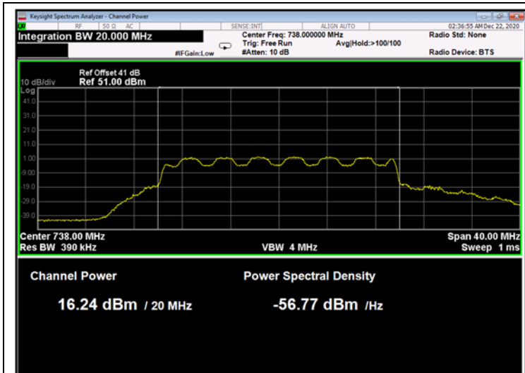
Figure 33: 16QAM 20MHz B.W.; 738.0MHz, 15kHz
