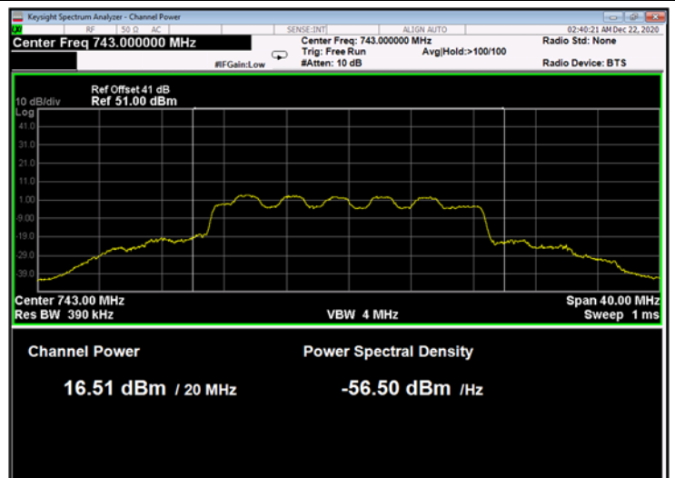
Figure 38: 16QAM 20MHz B.W.; 743.0MHz, 60kHz
