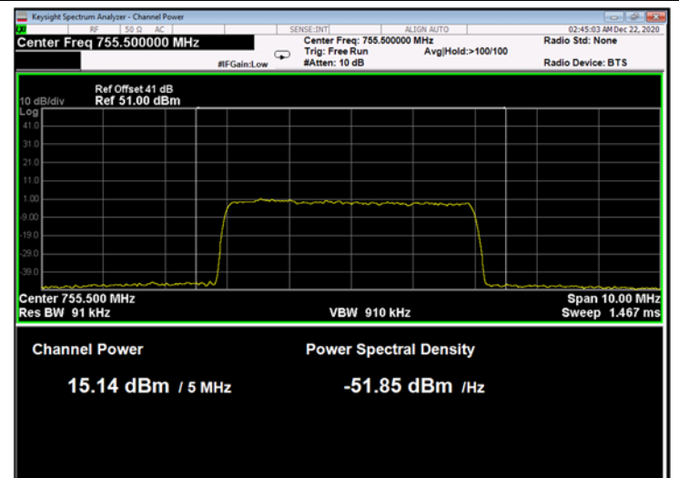
Figure 47: 64QAM 5MHz B.W.; 755.5MHz, 30kHz
