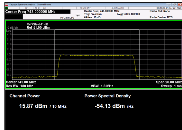
Figure 52: 64QAM 10MHz B.W.; 743.0MHz, 30kHz
