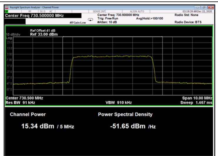
Figure 76: 256QAM 5MHz B.W.; 730.5MHz, 30kHz
