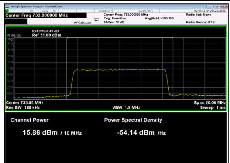
Figure 49: 64QAM 10MHz B.W.; 733.0MHz, 30kHz
