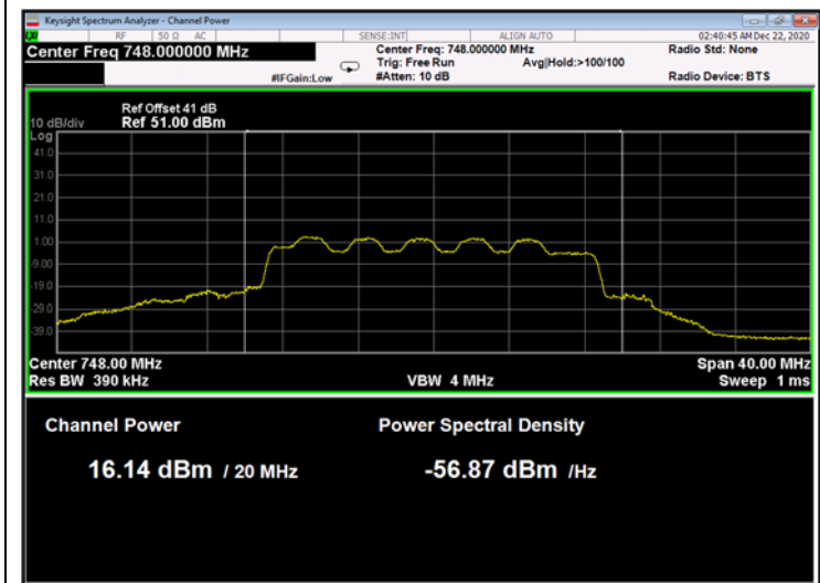
Figure 41: 16QAM 20MHz B.W.; 748.0MHz, 60kHz
