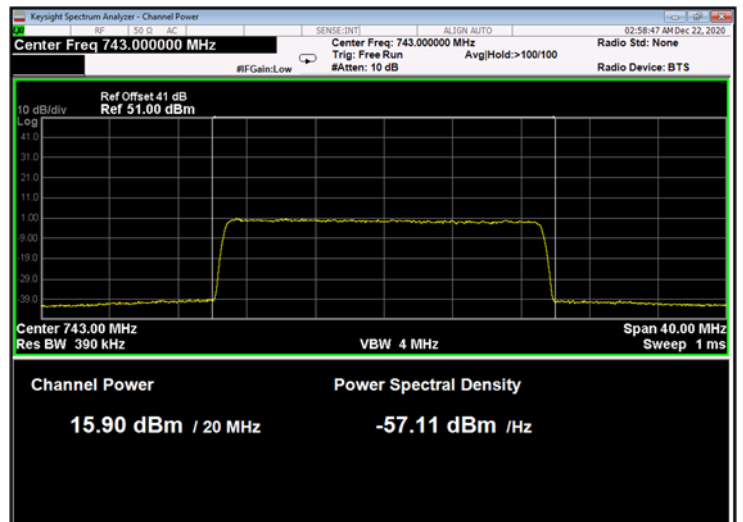
Figure 71: 64QAM 20MHz B.W.; 743.0MHz, 60kHz
