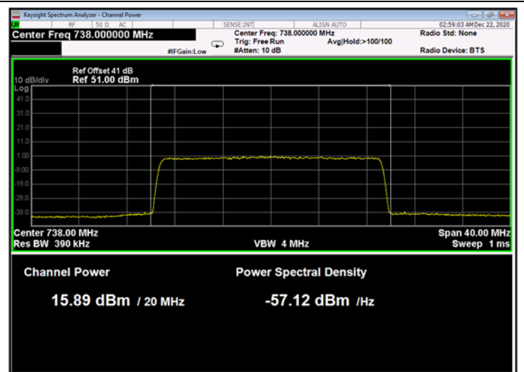
Figure 67: 64QAM 20MHz B.W.; 738.0MHz, 30kHz
