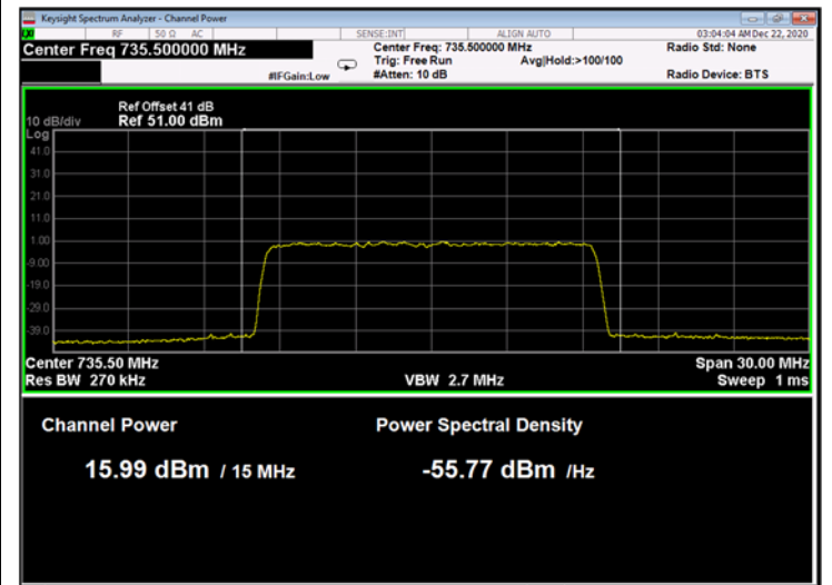
Figure 59: 64QAM 15MHz B.W.; 735.5MHz, 60kHz
