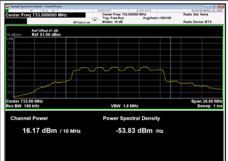
Figure 16: 16QAM 10MHz B.W.; 733.0MHz, 30kHz
