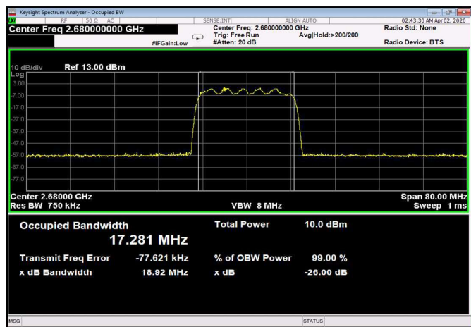
Figure 184: 16QAM 20MHz B.W.; 2680.0MHz, 60kHz Input
