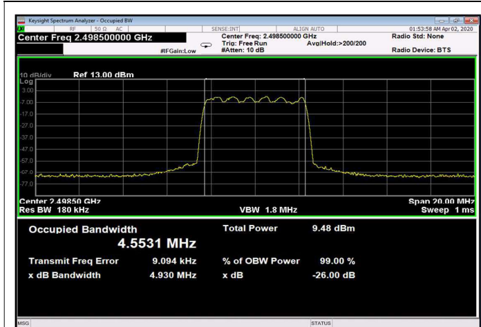
Figure 152: 16QAM 5MHz B.W.; 2498.5MHz, 15kHz Input
