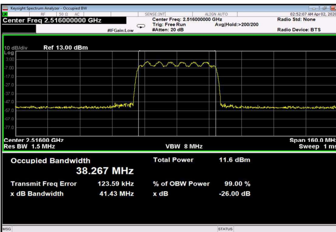
Figure 186: 16QAM 40MHz B.W.; 2516.0MHz, 30kHz Input
