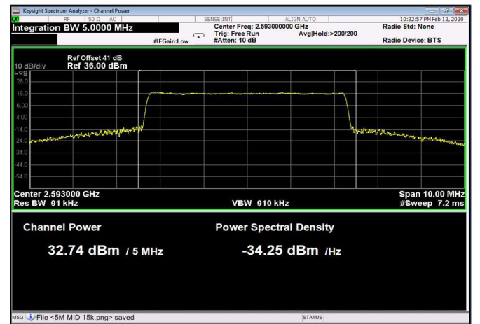
Figure 107: 256QAM 5MHz B.W.; 2593.0MHz, 15kHz
