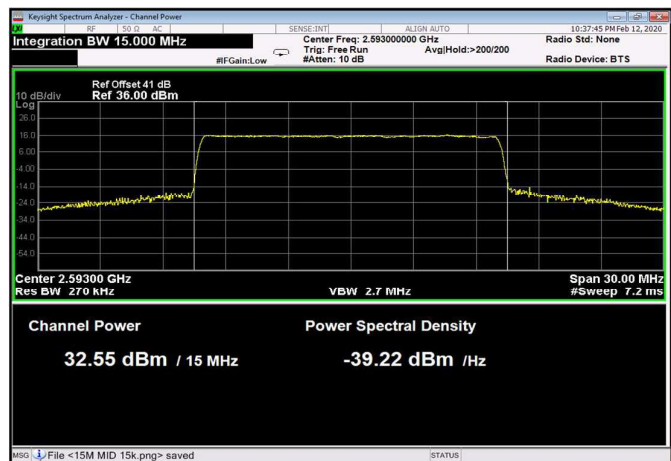
Figure 123: 256QAM 15MHz B.W.; 2593.0MHz, 30kHz
