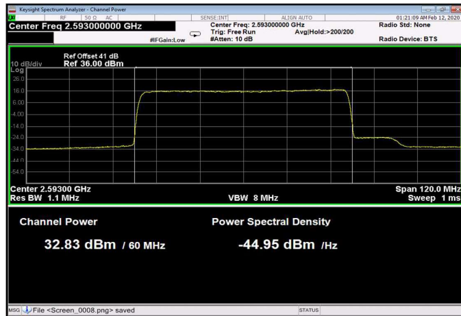
Figure 100: 64QAM 60MHz B.W.; 2593.0MHz, 30kHz
