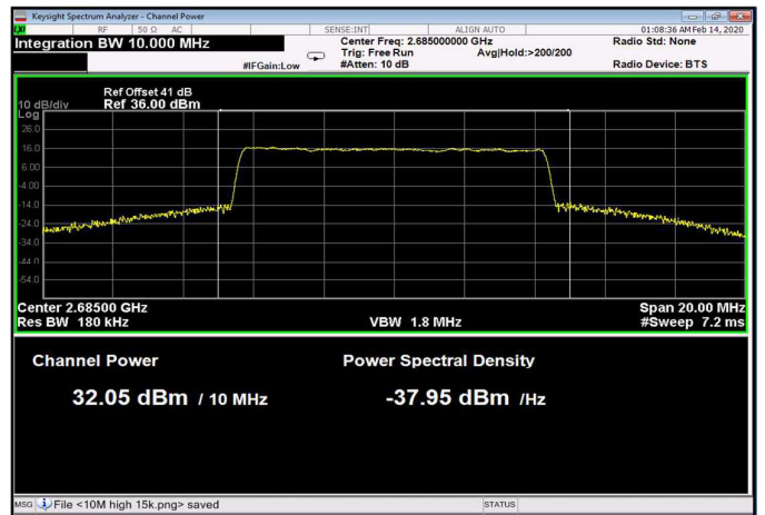
Figure 117: 256QAM 10MHz B.W.; 2685.0MHz, 30kHz
