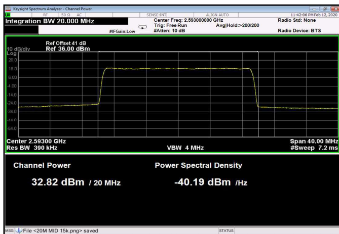
Figure 132: 256QAM 20MHz B.W.; 2593.0MHz, 30kHz
