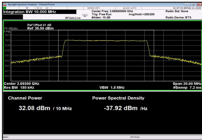
Figure 116: 256QAM 10MHz B.W.; 2685.0MHz, 15kHz
