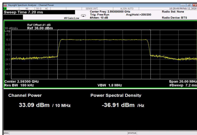
Figure 114: 256QAM 10MHz B.W.; 2593.0MHz, 30kHz
