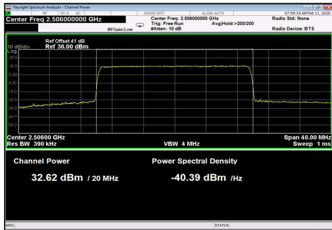
Figure 128: 256QAM 20MHz B.W.; 2506.0MHz, 15kHz
