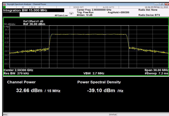
Figure 122: 256QAM 15MHz B.W.; 2593.0MHz, 15kHz
