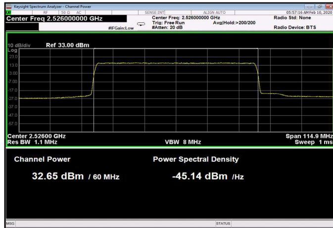
Figure 98: 64QAM 60MHz B.W.; 2526.0MHz, 30kHz
