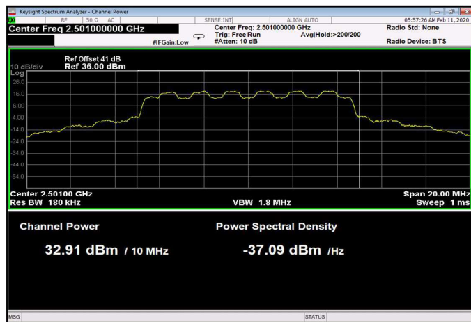
Figure 14: 16QAM 10MHz B.W.; 2501.0MHz, 15kHz
