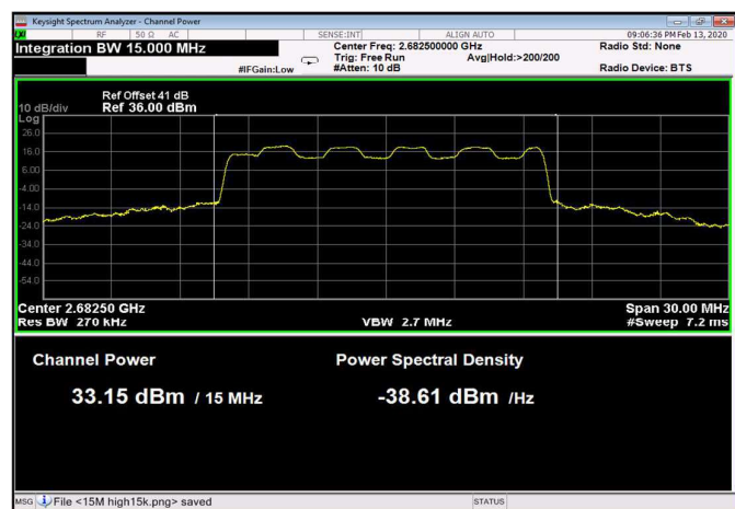
Figure 30: 16QAM 15MHz B.W.; 2682.5MHz, 30kHz
