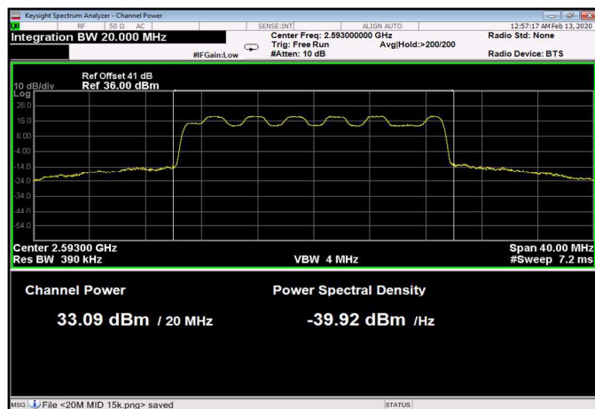
Figure 36: 16QAM 20MHz B.W.; 2593.0MHz, 30kHz
