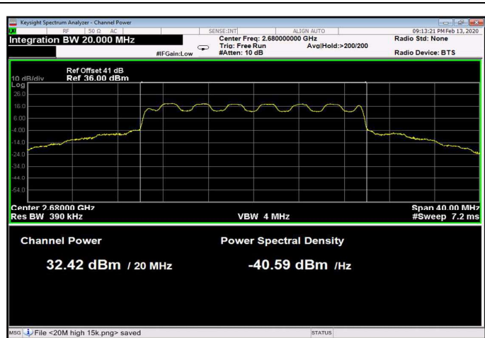
Figure 39: 16QAM 20MHz B.W.; 2680.0MHz, 30kHz
