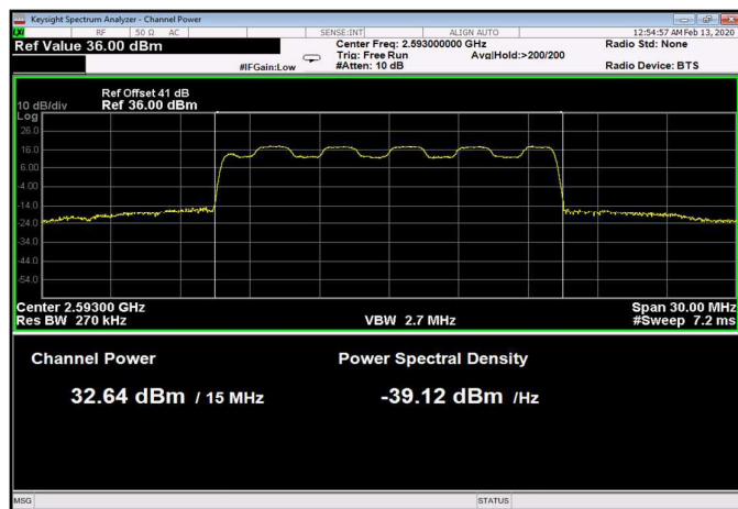
Figure 28: 16QAM 15MHz B.W.; 2593.0MHz, 60kHz
