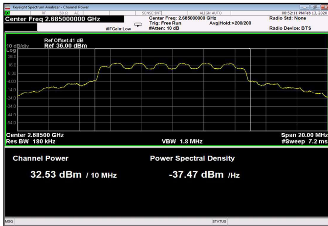
Figure 20: 16QAM 10MHz B.W.; 2685.0MHz, 15kHz
