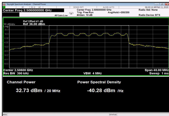
Figure 32: 16QAM 20MHz B.W.; 2506.0MHz, 15 kHz
