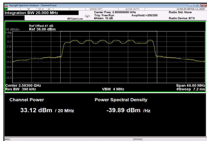
Figure 35: 16QAM 20MHz B.W.; 2593.0MHz, 15kHz
