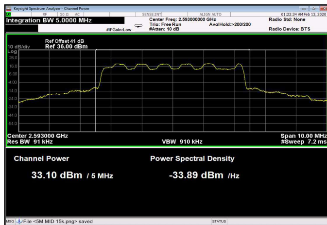
Figure 10: 16QAM 5MHz B.W.; 2593.0MHz, 15kHz
