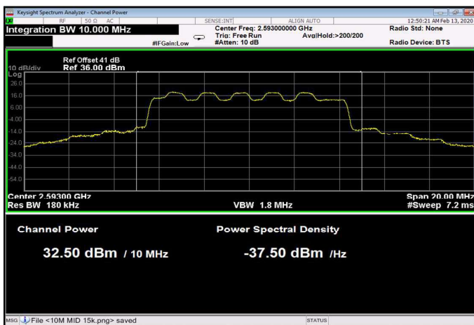
Figure 18: 16QAM 10MHz B.W.; 2593.0MHz, 30kHz
