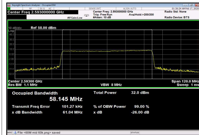
Figure 436: 256QAM 60MHz B.W.; 2593.0MHz, 30kHz Output
