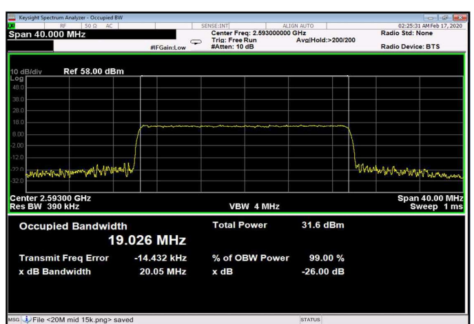
Figure 419: 256QAM 20MHz B.W.; 2593.0MHz, 15kHz Output
