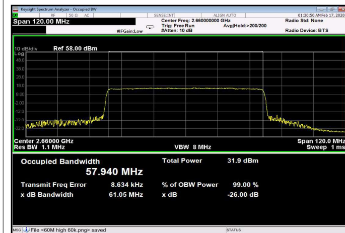
Figure 438: 256QAM 60MHz B.W.; 2660.0MHz, 30kHz Output
