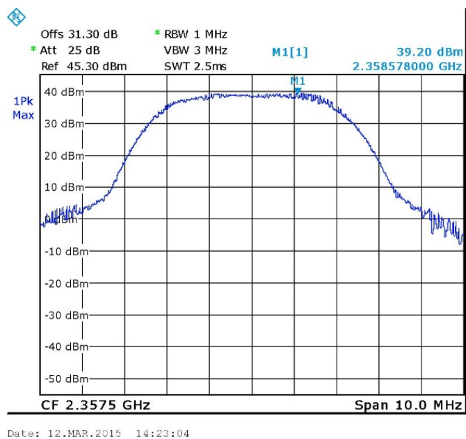
Figure 20. — 2357.5MHz- W-CDMA
