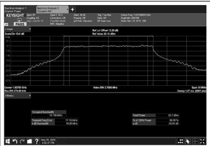
Figure 254: 64QAM 15MHz B.W.; 1937.5MHz, 30kHz Output
