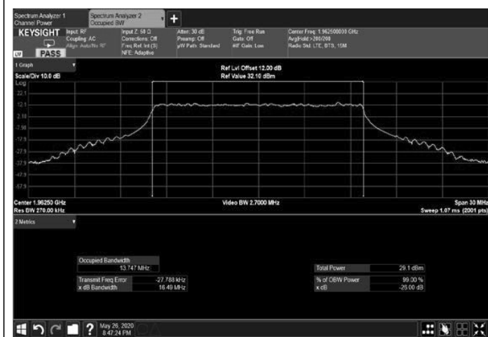
Figure 257: 64QAM 15MHz B.W.; 1962.5MHz, 30kHz Output
