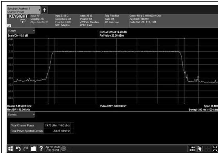
Figure 145: 64QAM 10MHz B.W.; 2115.0MHz, 15kHz
