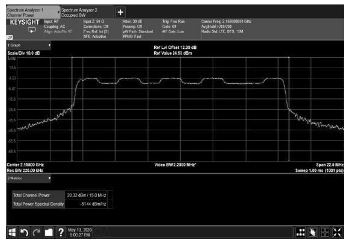
Figure 124: 16QAM 15MHz B.W.; 2155.0MHz, 15kHz
