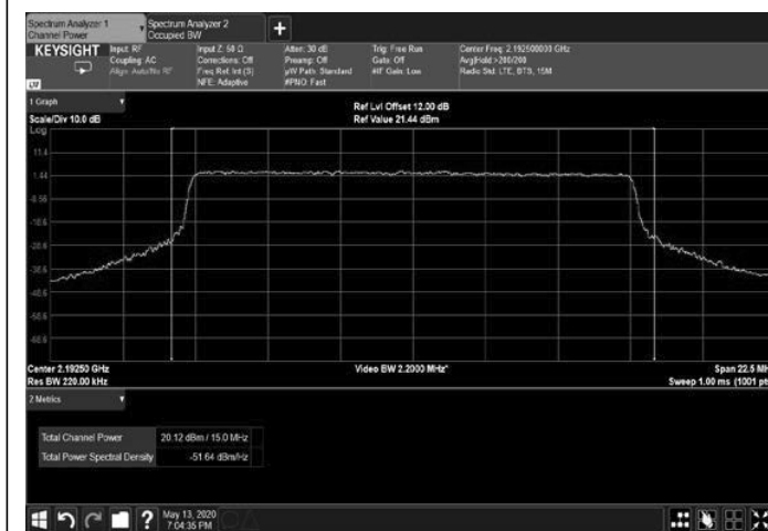
Figure 161: 64QAM 15MHz B.W.; 2192.5MHz, 30kHz
