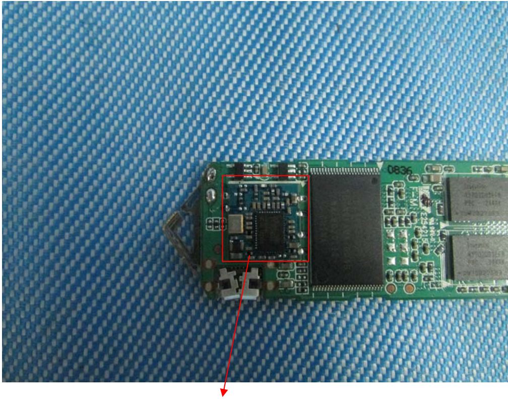
RF module
