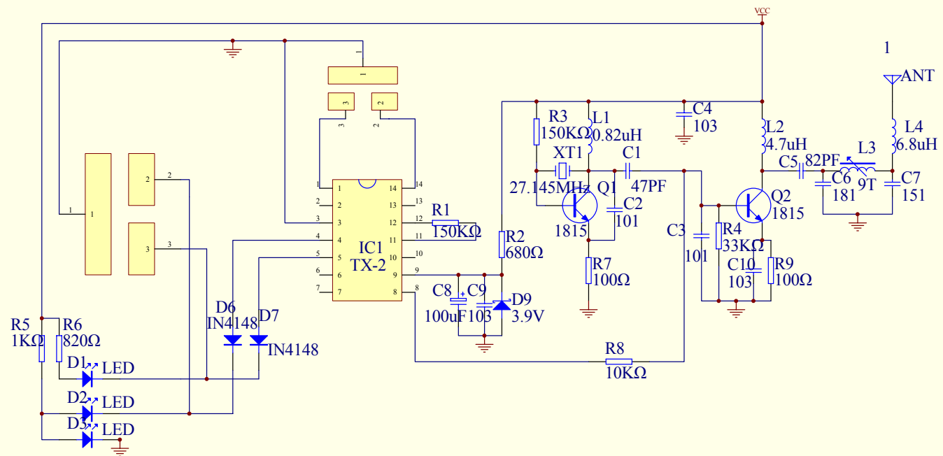
17039 27MHz发射电路图
