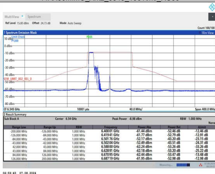
11AX80MIMO_Ant2_6545_242Tone_RU61
