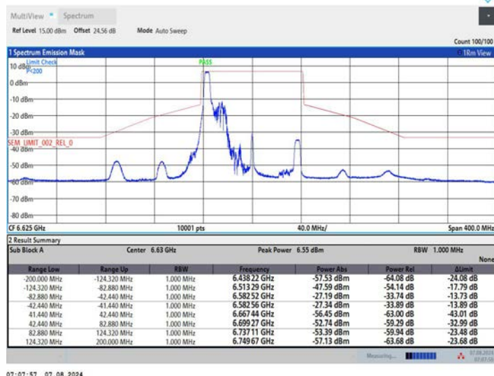
11AX80MIMO_Ant2_6625_106Tone_RU53
