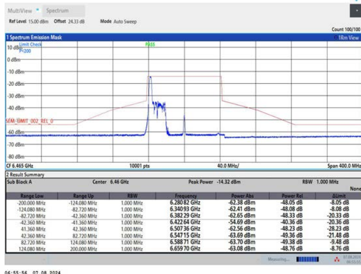
11AX80MIMO_Ant1_6465_52Tone_RU37
