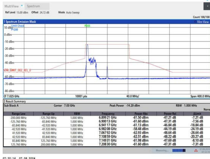
11AX80MIMO_Ant1_7025_52Tone_RU37
