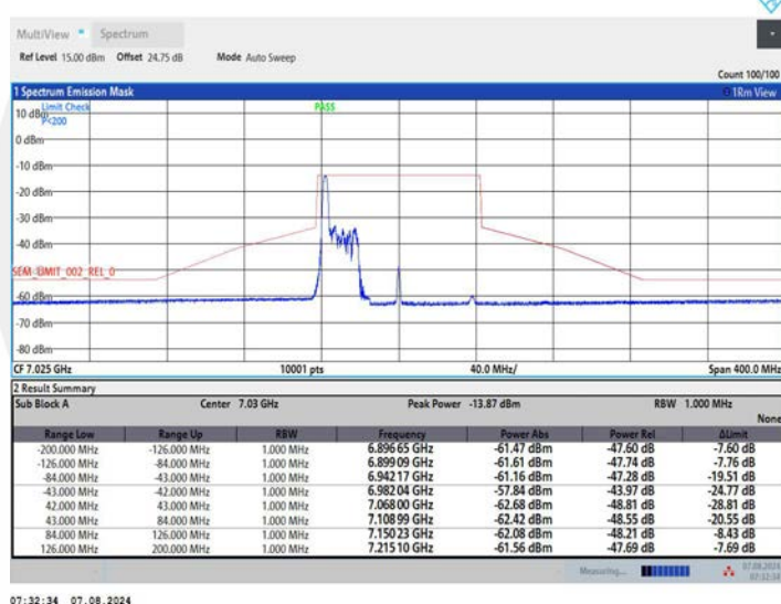
11AX80MIMO_Ant2_7025_52Tone_RU37
