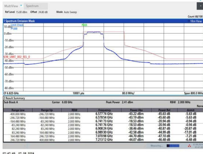
11AX160MIMO_Ant2_6825_996Tone_RU67
