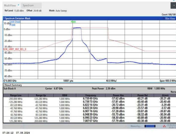
11AX80MIMO_Ant1_6865_484Tone_RU65
