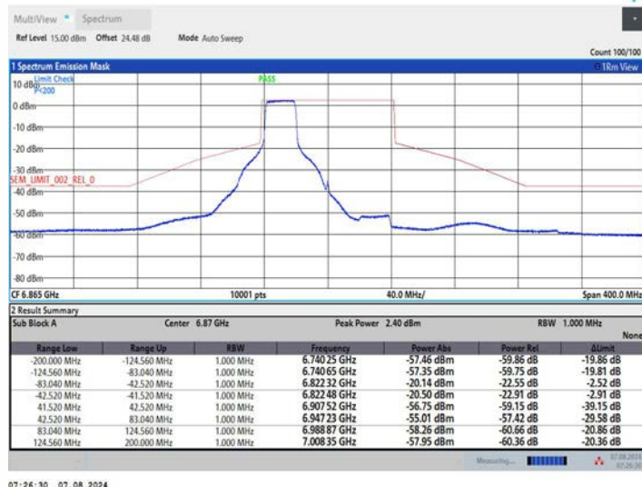
11AX80MIMO_Ant2_6865_484Tone_RU65
