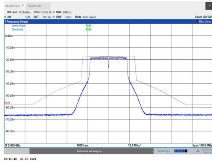
11N20MIMO_Ant2_5955
