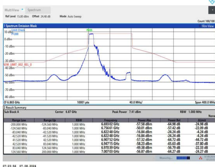
11AX80MIMO_Ant2_6865_242Tone_RU61
