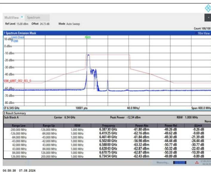
11AX80MIMO_Ant2_6545_106Tone_RU53
