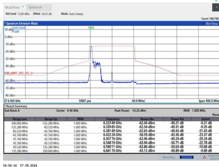
11AX80MIMO_Ant2_6465_52Tone_RU37
