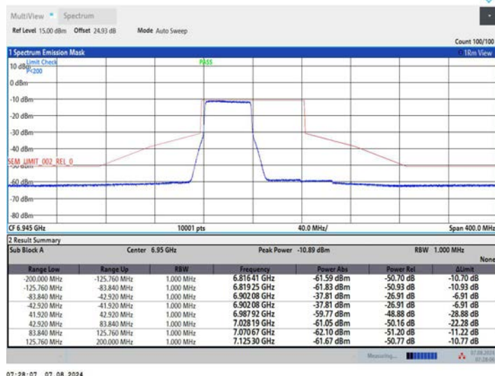
11AX80MIMO_Ant2_6945_26Tone_RU0
