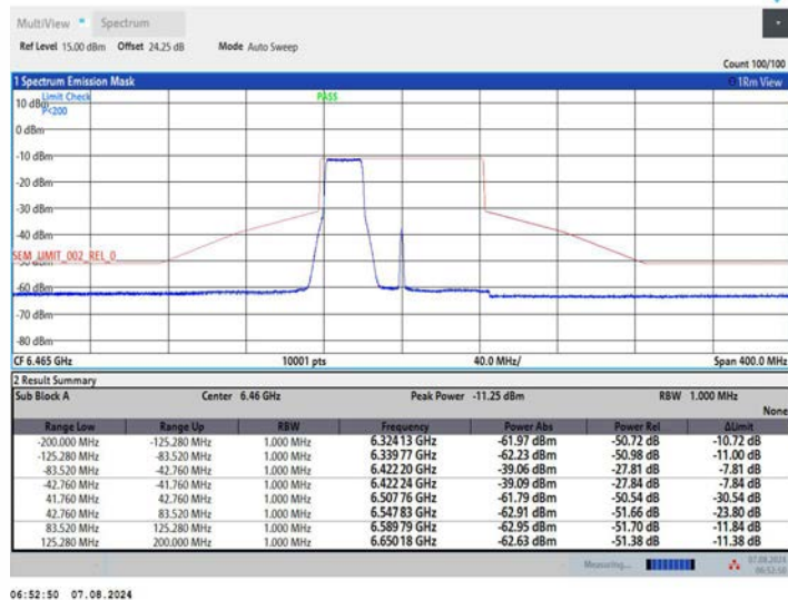
11AX80MIMO_Ant2_6465_484Tone_RU65
