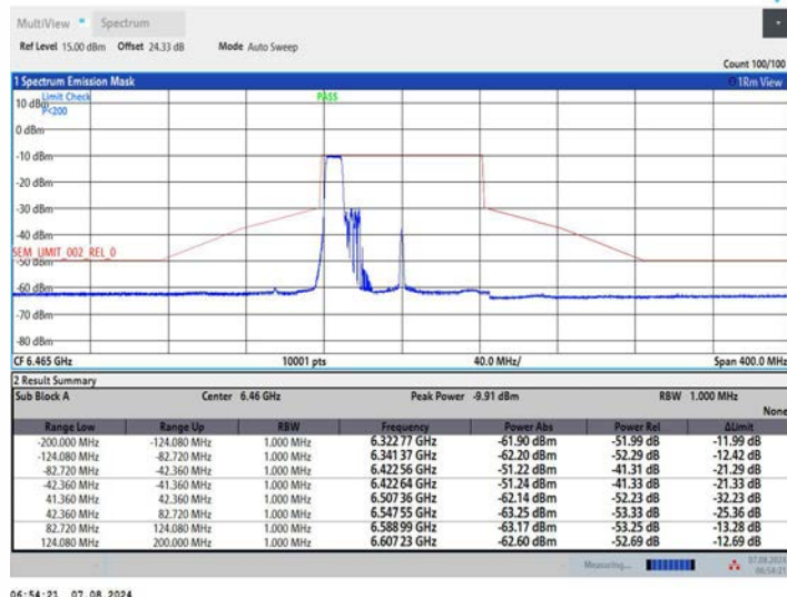
11AX80MIMO_Ant1_6465_242Tone_RU61
