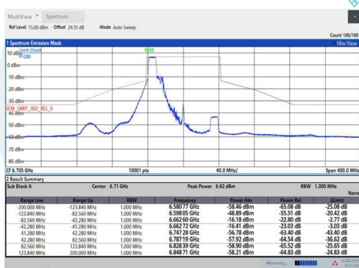
11AX80MIMO_Ant2_6705_242Tone_RU61
