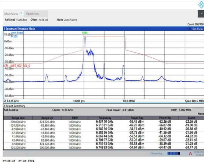
11AX80MIMO_Ant2_6625_52Tone_RU37
