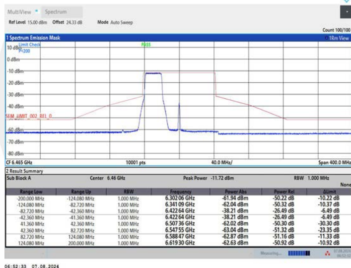
11AX80MIMO_Ant1_6465_484Tone_RU65
