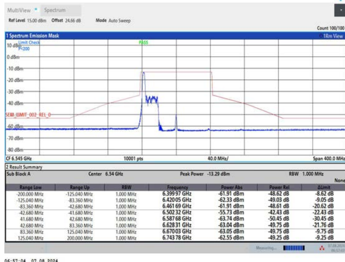
11AX80MIMO_Ant1_6545_52Tone_RU37
