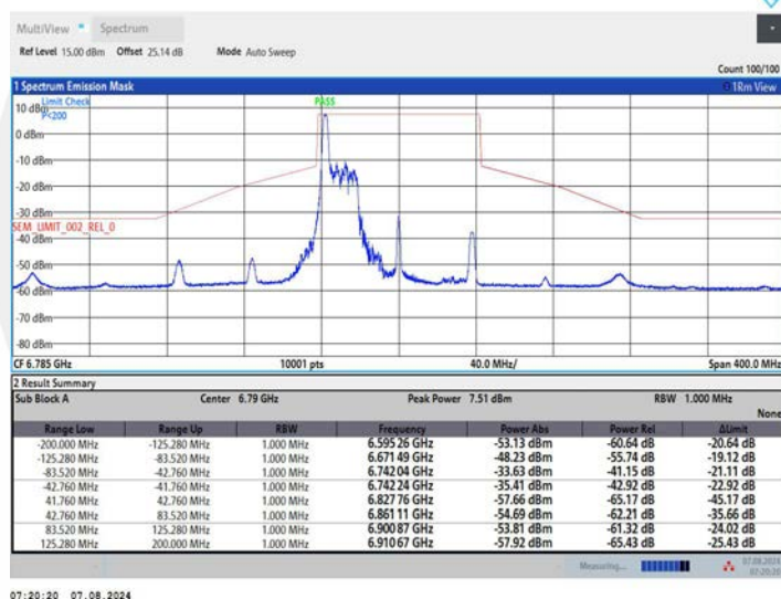
11AX80MIMO_Ant2_6785_52Tone_RU37
