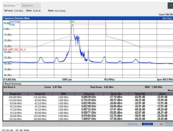
11AX80MIMO_Ant2_6865_106Tone_RU53
