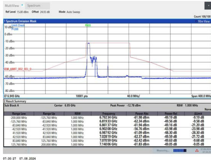
11AX80MIMO_Ant1_6945_106Tone_RU53
