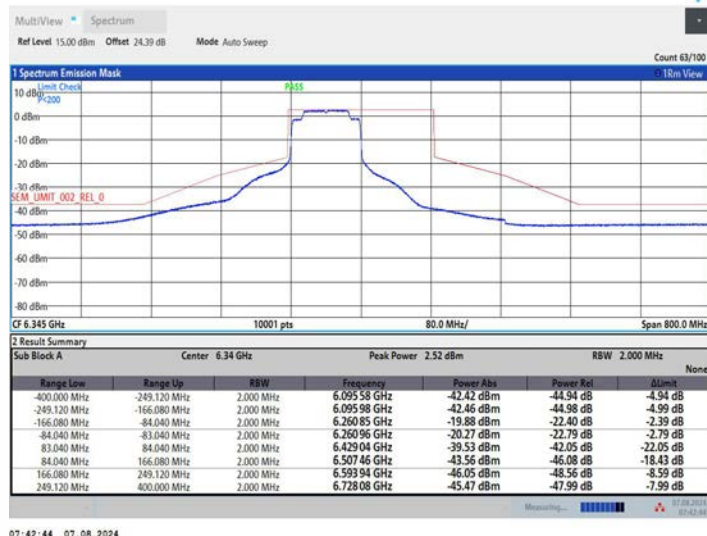
11AX160MIMO_Ant2_6345_996Tone_RU67
