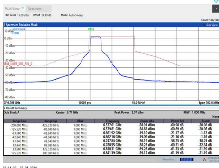
11AX80MIMO_Ant1_6705_484Tone_RU65
