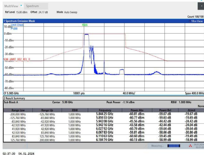
11AX80MIMO_Ant2_5985_242Tone_RU61
