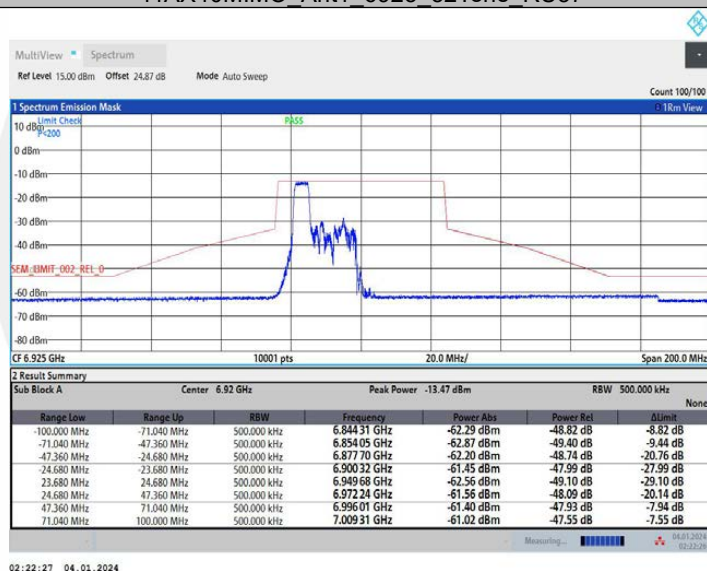
11AX40MIMO Ant1 6925 106Tone RU53
