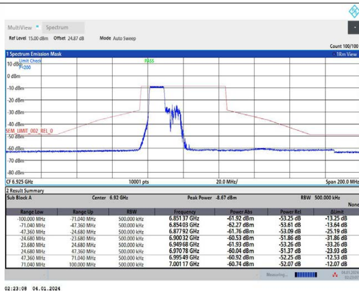
11AX40MIMO_Ant1_6925_242Tone_RU61
