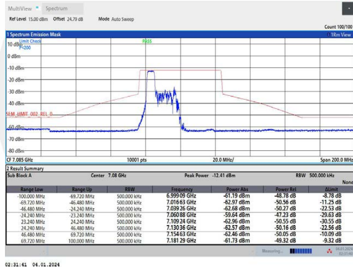
11AX40MIMO Ant1 7085 106Tone RU53
