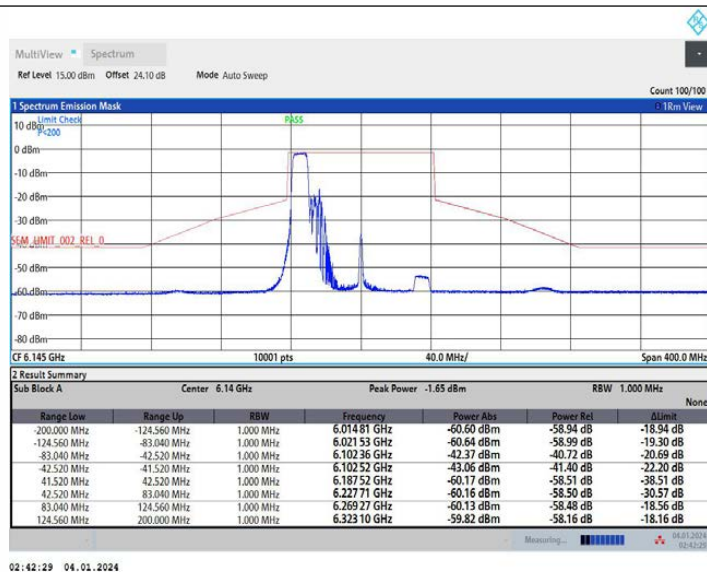
11AX80MIMO_Ant2_6145_242Tone_RU61
