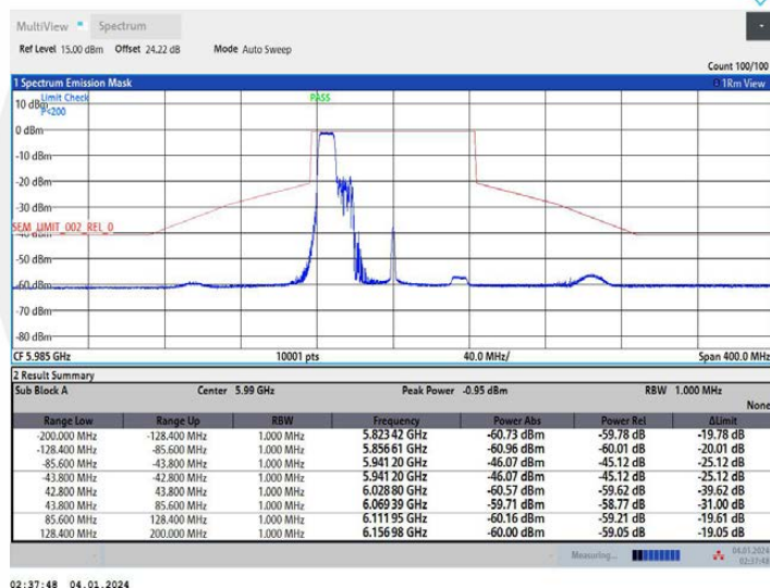
11AX80MIMO_Ant1_5985_242Tone_RU61
