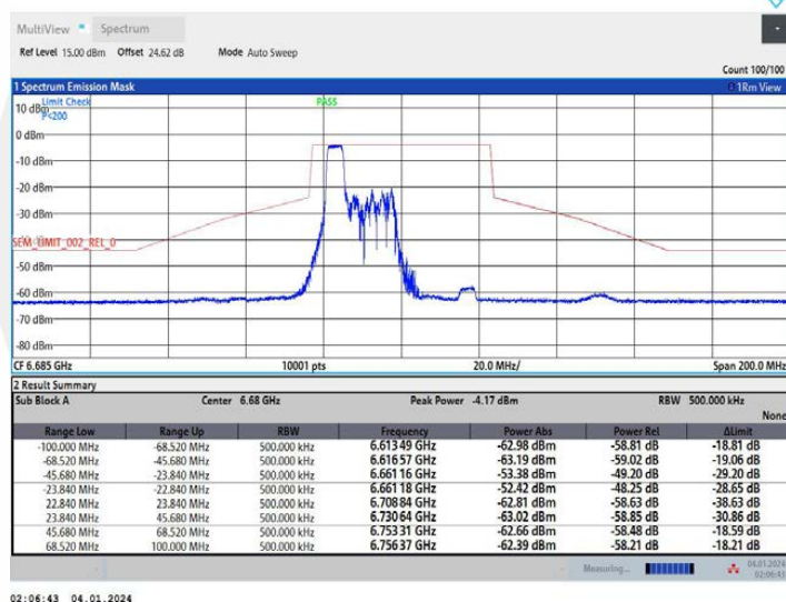
11AX40MIMO Ant1 6685 106Tone RU53
