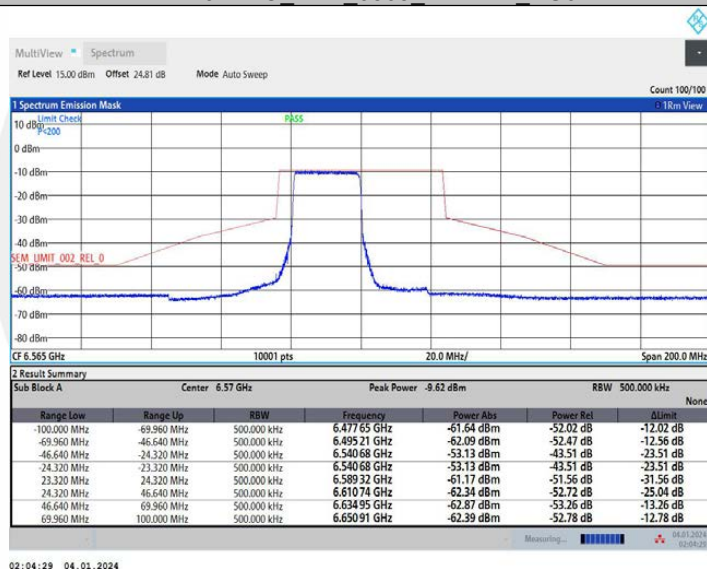
11AX40MIMO_Ant1_6565_26Tone_RU0
