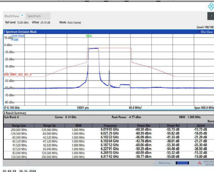
11AX80MIMO_Ant2_6145_484Tone_RU65
