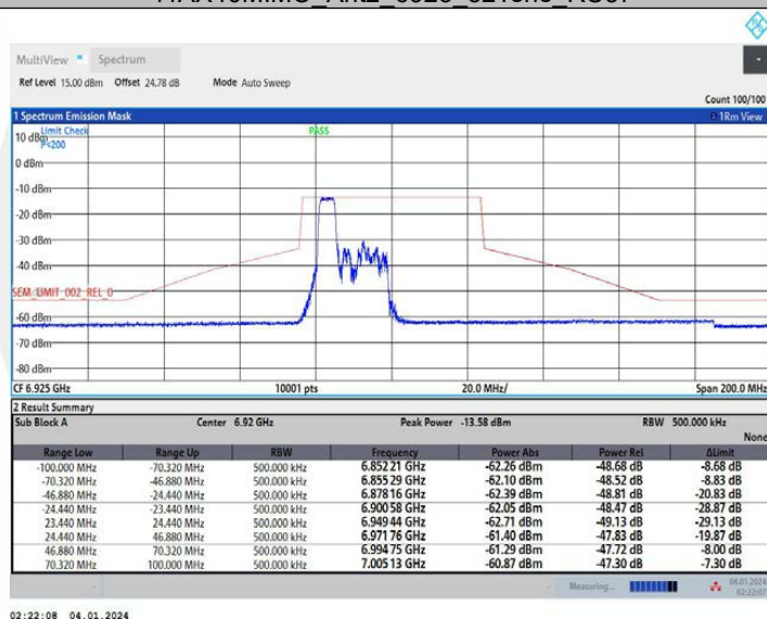
11AX40MIMO_Ant2_6925_106Tone_RU53
