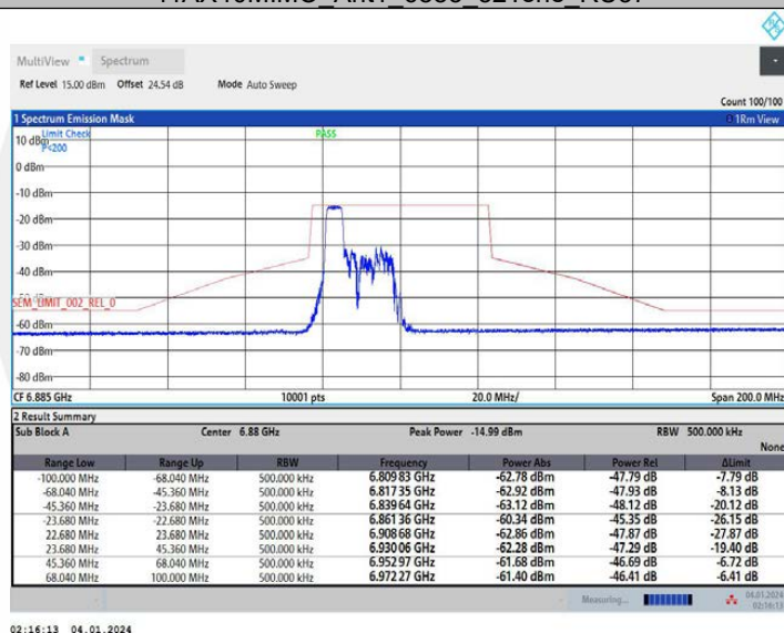
11AX40MIMO Ant1 6885 106Tone RU53
