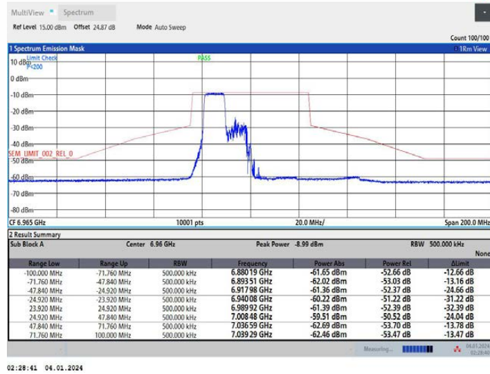
11AX40MIMO Ant1 6965 242Tone RU61
