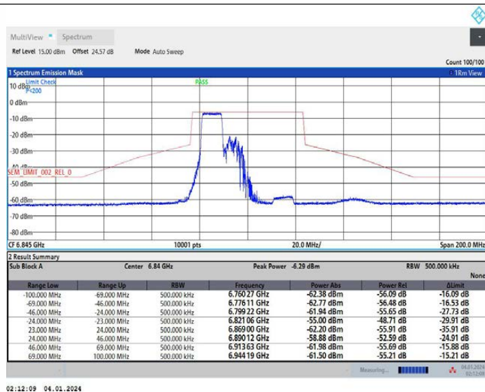
11AX40MIMO_Ant2_6845_242Tone_RU61
