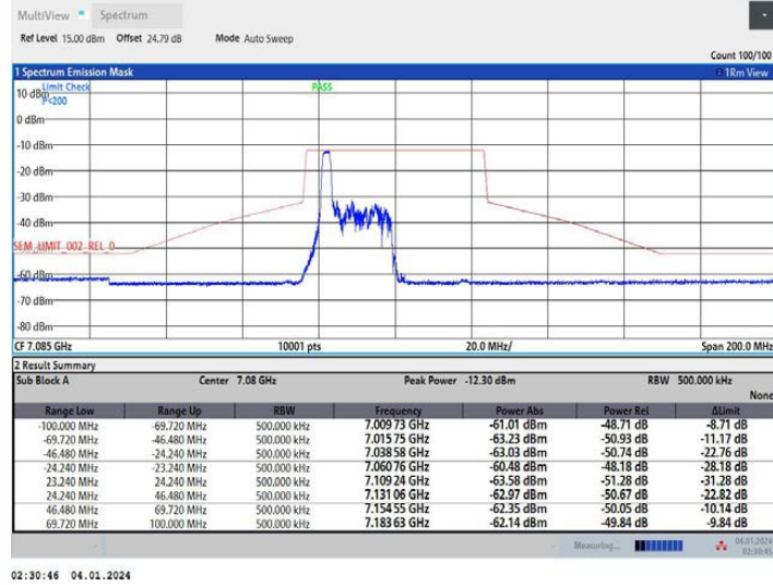
11AX40MIMO Ant1 7085 52Tone RU37
