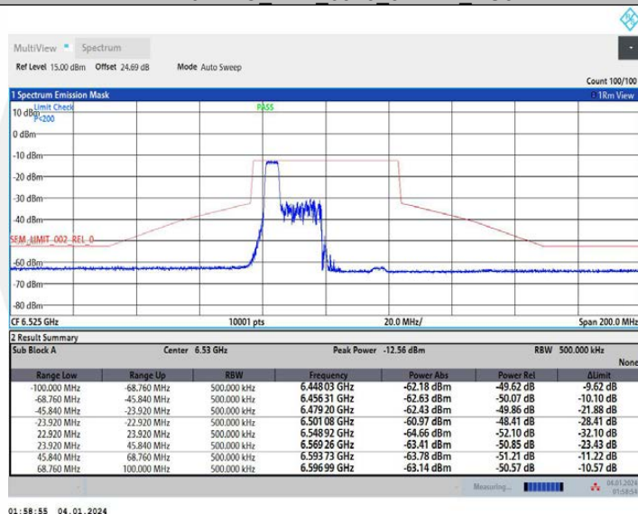
11AX40MIMO Ant1 6525 106Tone RU53
