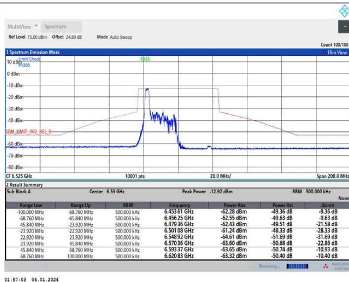
11AX40MIMO Ant1 6525 52Tone RU37
