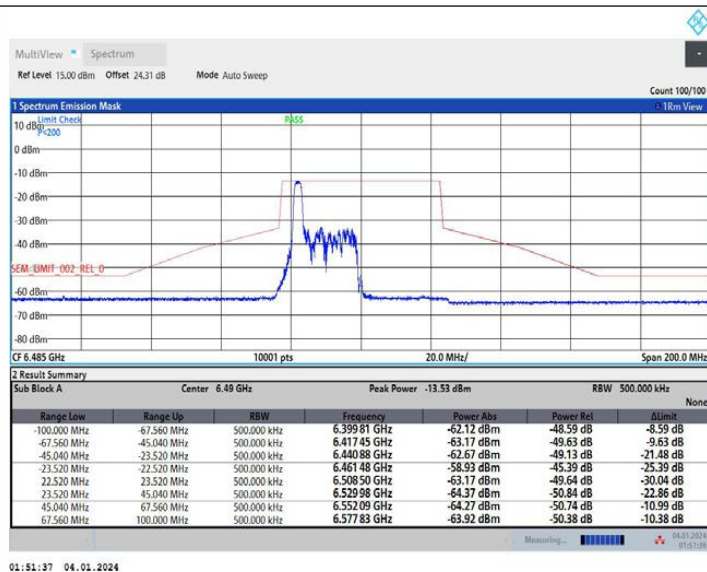
11AX40MIMO Ant1 6485 52Tone RU37
