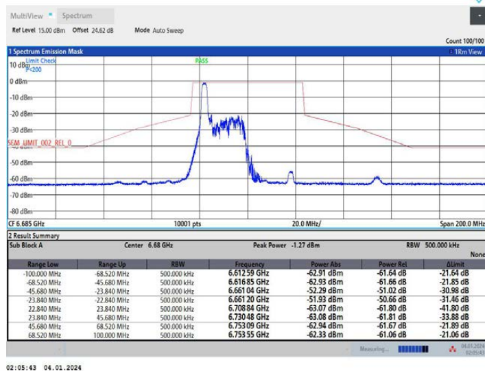
11AX40MIMO Ant1 6685 52Tone RU37
