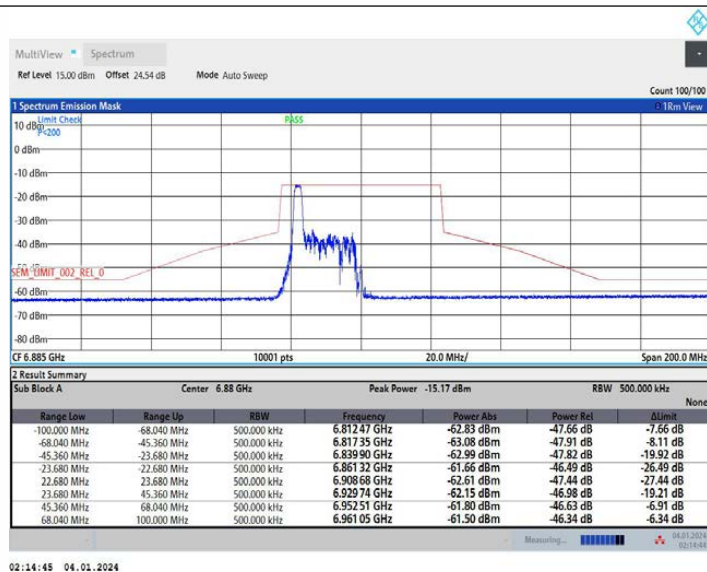
11AX40MIMO Ant1 6885 52Tone RU37
