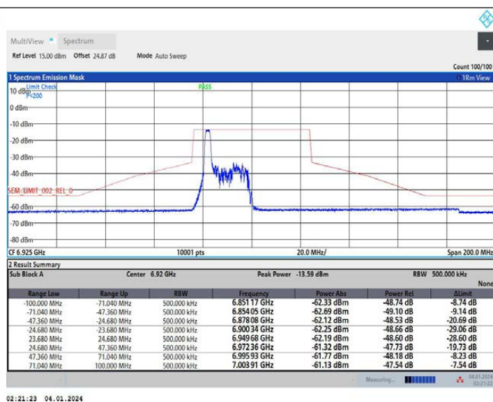
11AX40MIMO Ant1 6925 52Tone RU37
