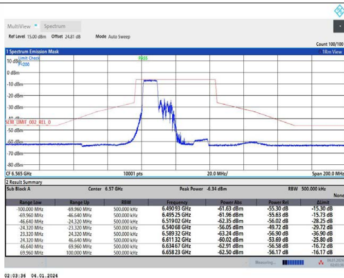
11AX40MIMO_Ant2_6565_242Tone_RU61
