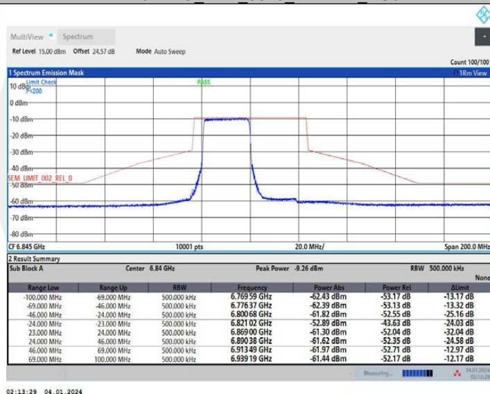
11AX40MIMO_Ant1_6845_26Tone_RU0
