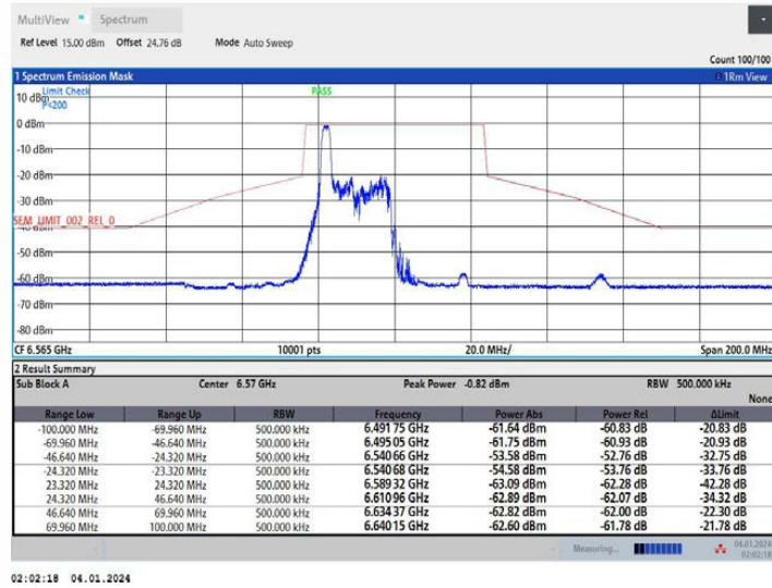
11AX40MIMO Ant1 6565 52Tone RU37
