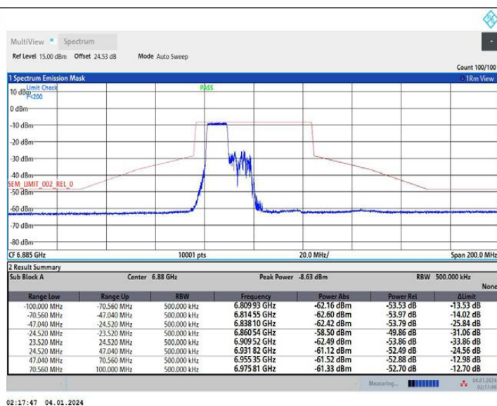
11AX40MIMO_Ant2_6885_242Tone_RU61
