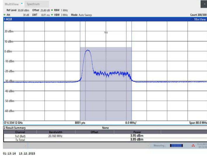
11AX40MIMO_Ant1_6565_52Tone_RU37
