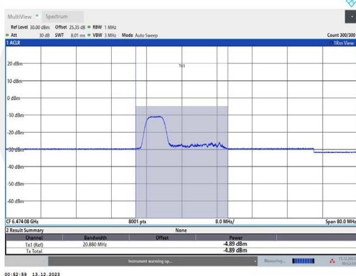
11AX40MIMO_Ant1_6485_106Tone_RU53
