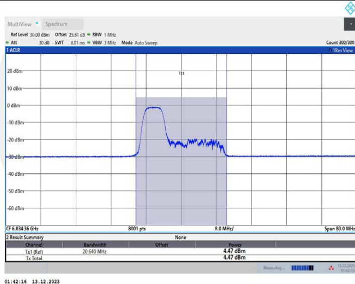
11AX40MIMO_Ant2_6845_106Tone_RU53
