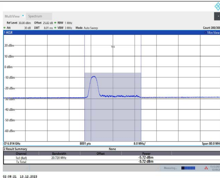
11AX40MIMO_Ant2_6925_52Tone_RU37
