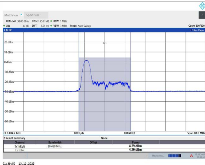
11AX40MIMO_Ant2_6845_52Tone_RU37
