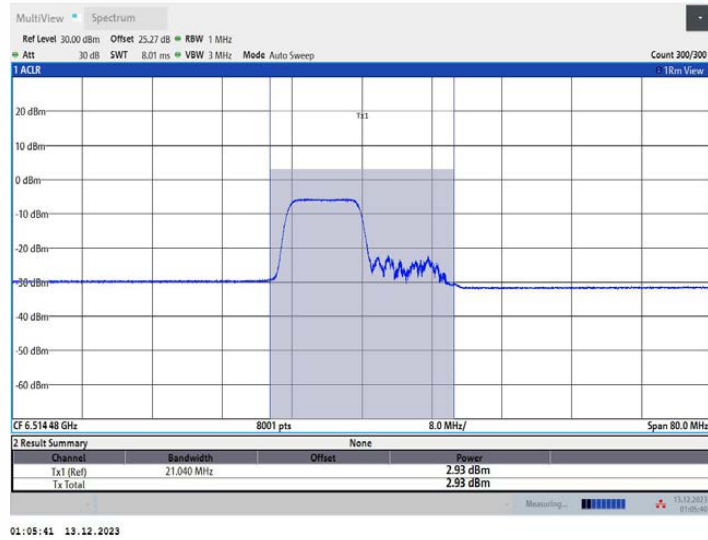
11AX40MIMO_Ant1_6525_242Tone_RU61
