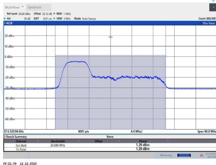
11AX20MIMO_Ant2_6535_106Tone_RU53
