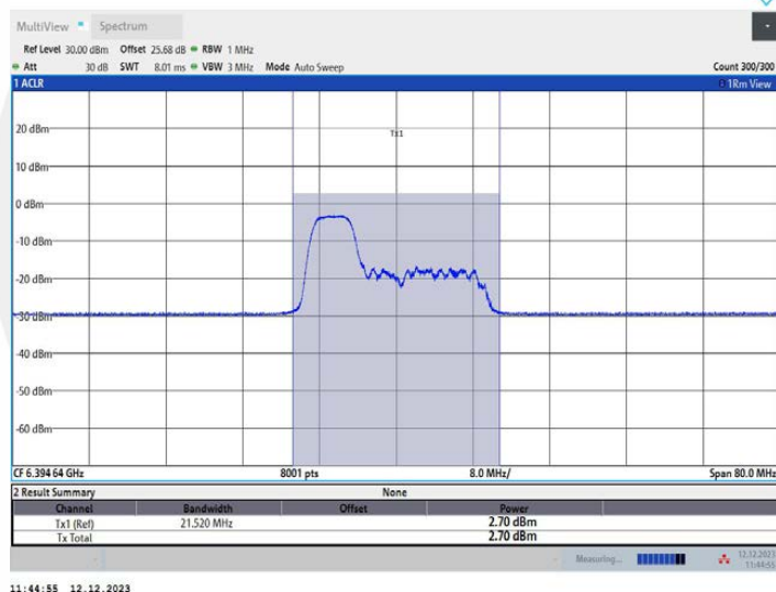
11AX40MIMO_Ant2_6405_106Tone_RU53
