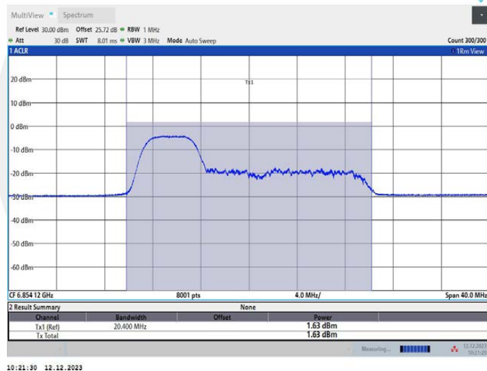
11AX20MIMO_Ant2_6855_106Tone_RU53
