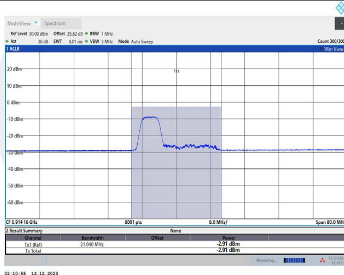
11AX40MIMO_Ant2_6925_106Tone_RU53
