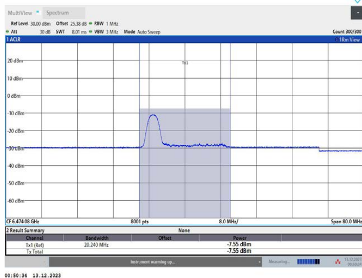
11AX40MIMO_Ant1_6485_52Tone_RU37
