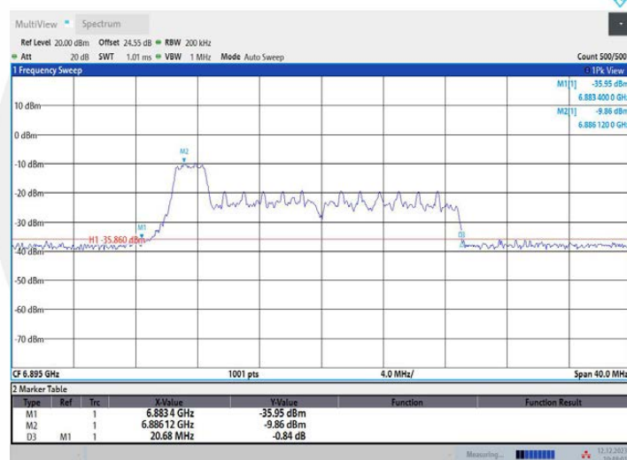
11AX20MIMO_Ant1_6895_52Tone_RU37
