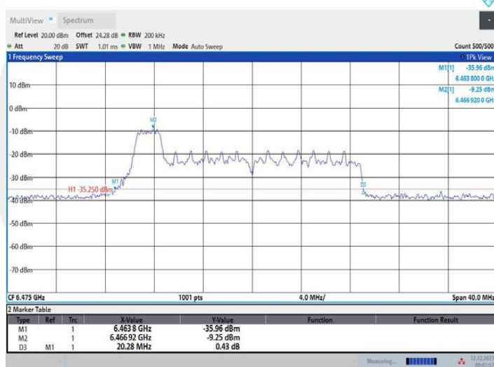
11AX20MIMO_Ant1_6475_52Tone_RU37
