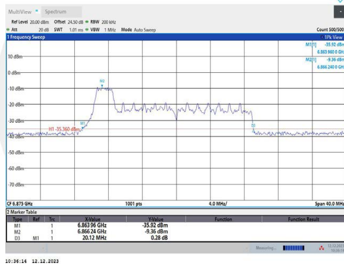
11AX20MIMO_Ant1_6875_52Tone_RU37
