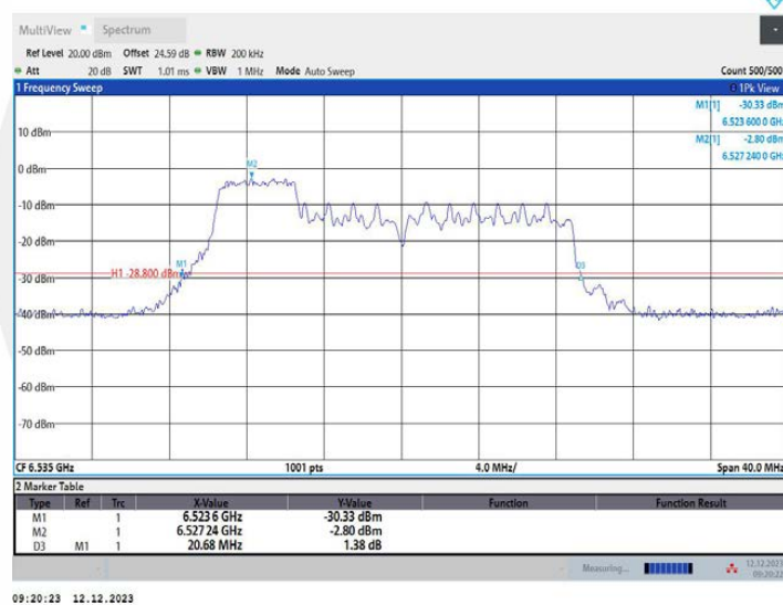
11AX20MIMO_Ant2_6535_106Tone_RU53
