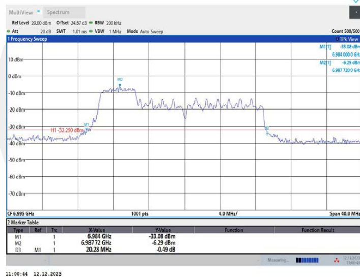
11AX20MIMO_Ant2_6995_106Tone_RU53
