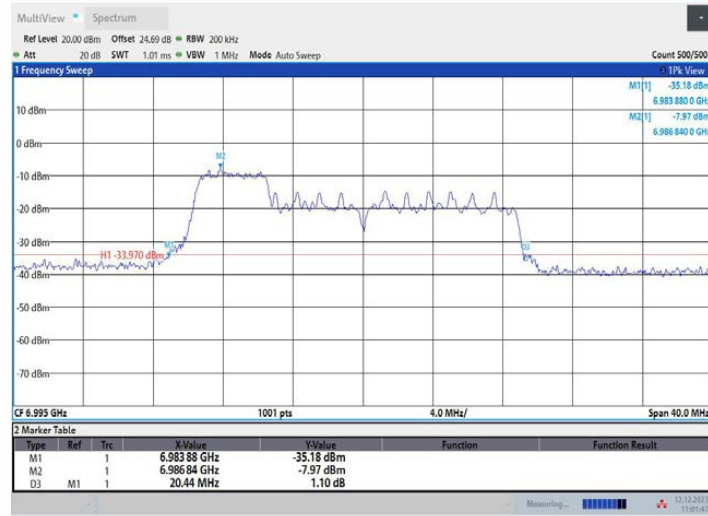
11AX20MIMO_Ant1_6995_106Tone_RU53
