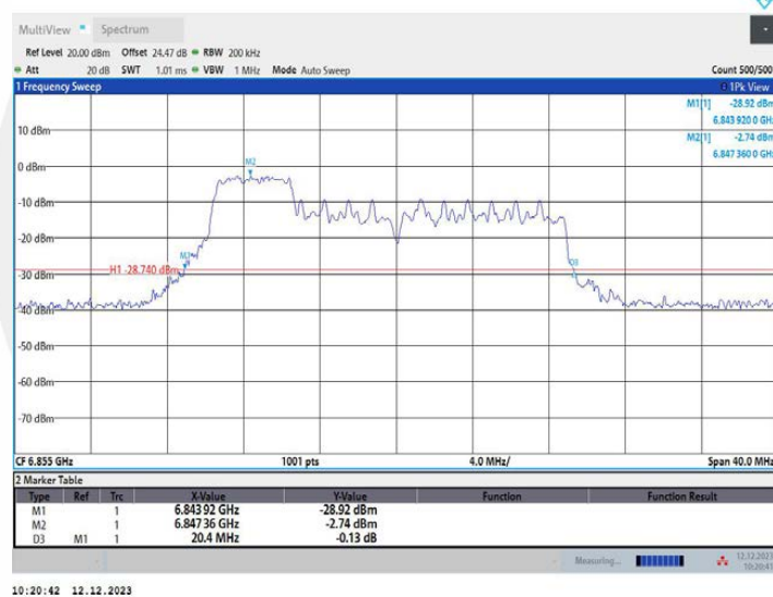
11AX20MIMO_Ant2_6855_106Tone_RU53
