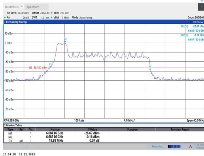
11AX20MIMO_Ant1_6695_52Tone_RU37
