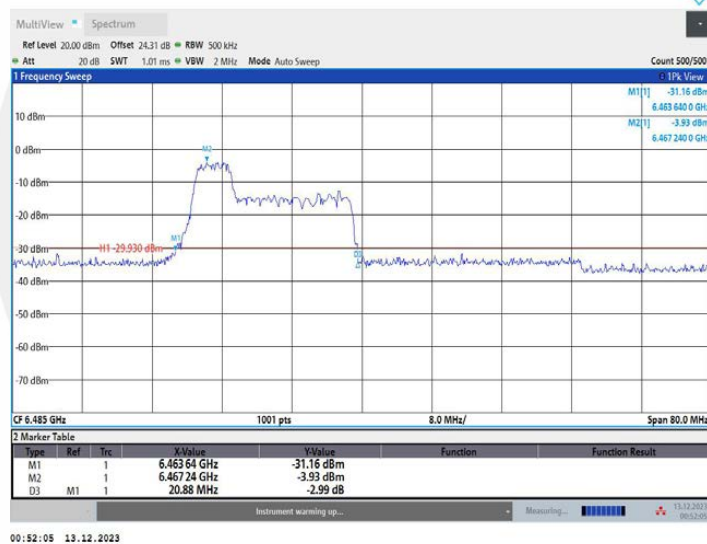
11AX40MIMO_Ant1_6485_106Tone_RU53
