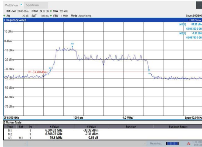
11AX20MIMO_Ant1_6515_106Tone_RU53
