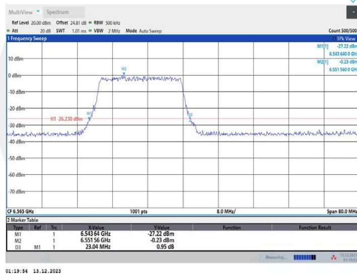
11AX40MIMO_Ant1_6565_26Tone_RU0
