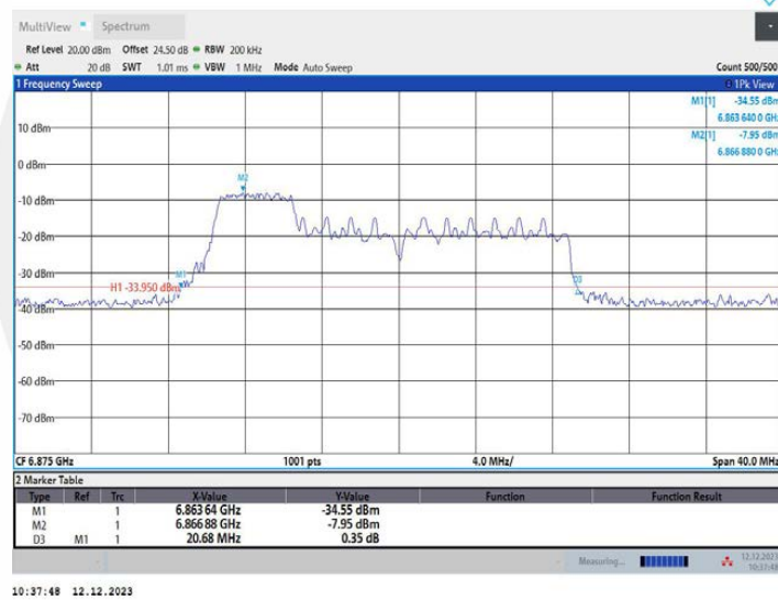
11AX20MIMO_Ant2_6875_106Tone_RU53
