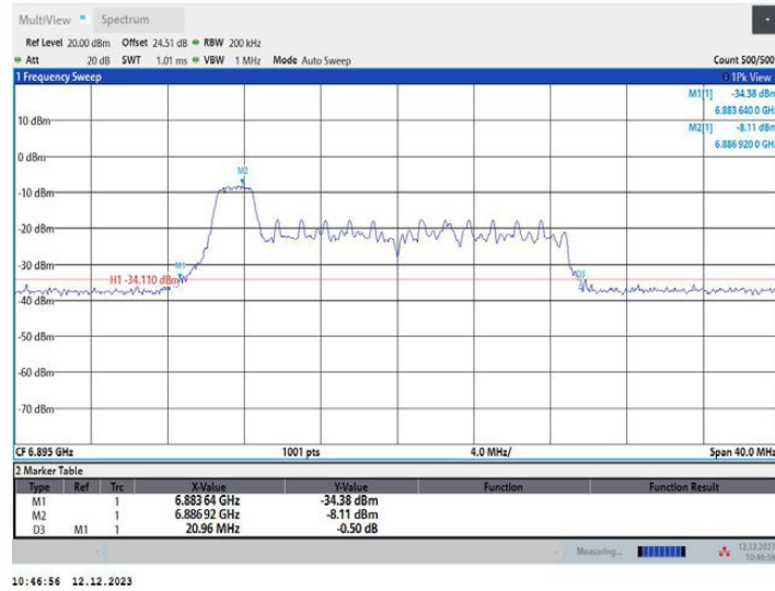
11AX20MIMO_Ant2_6895_52Tone_RU37
