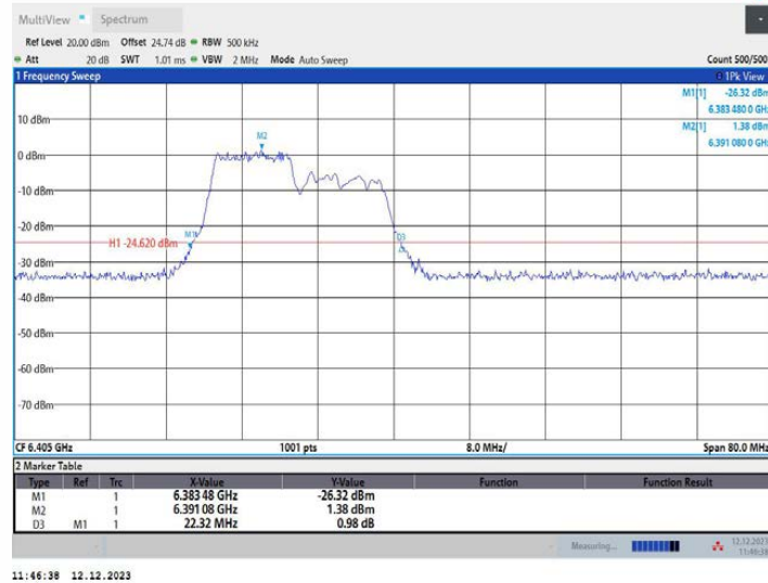
11AX40MIMO_Ant2_6405_242Tone_RU61
