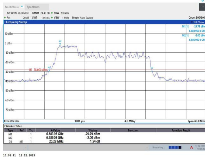
11AX20MIMO_Ant2_6695_106Tone_RU53
