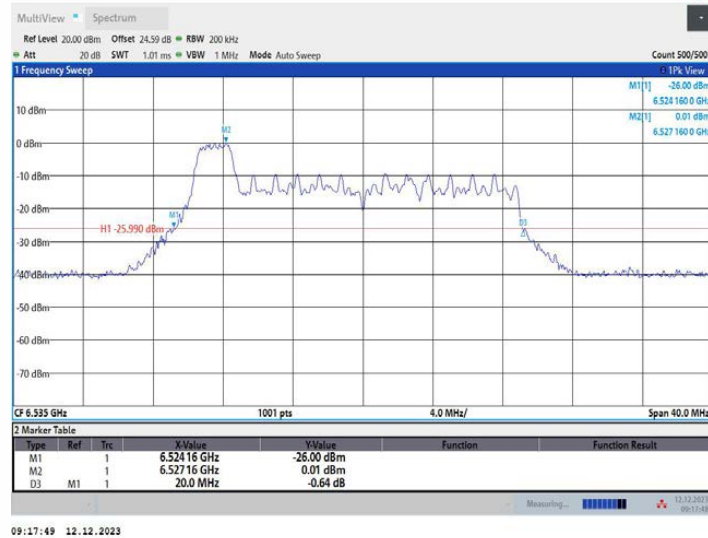
11AX20MIMO_Ant2_6535_52Tone_RU37
