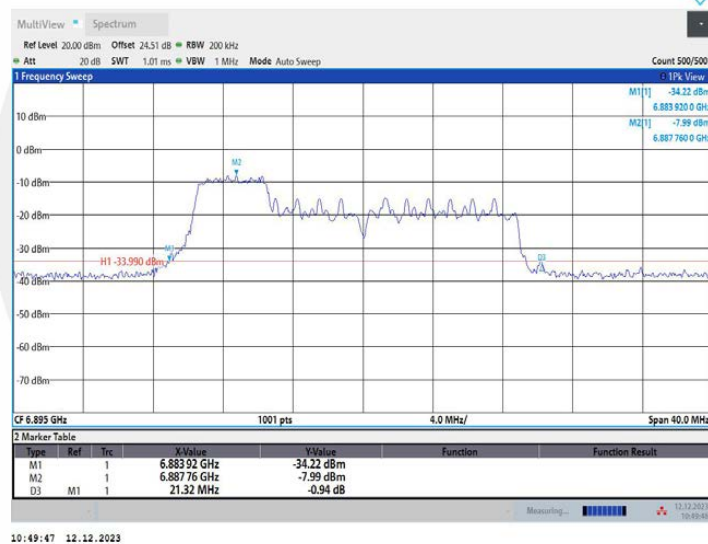
11AX20MIMO_Ant2_6895_106Tone_RU53
