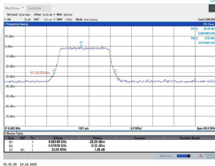
11AX40MIMO_Ant1_6685_26Tone_RU0
