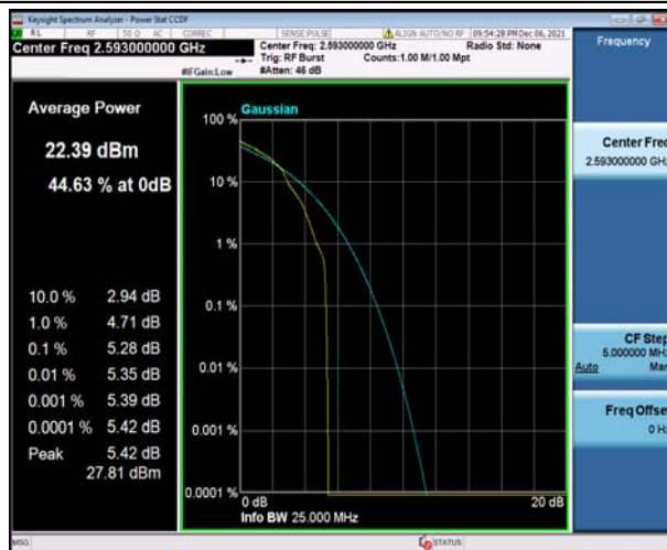
Band41-20MHz-16QAM-41490-1RB#0
