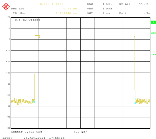
2-DH5
