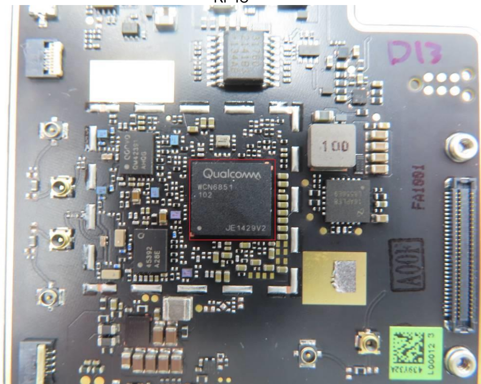
RF IC
