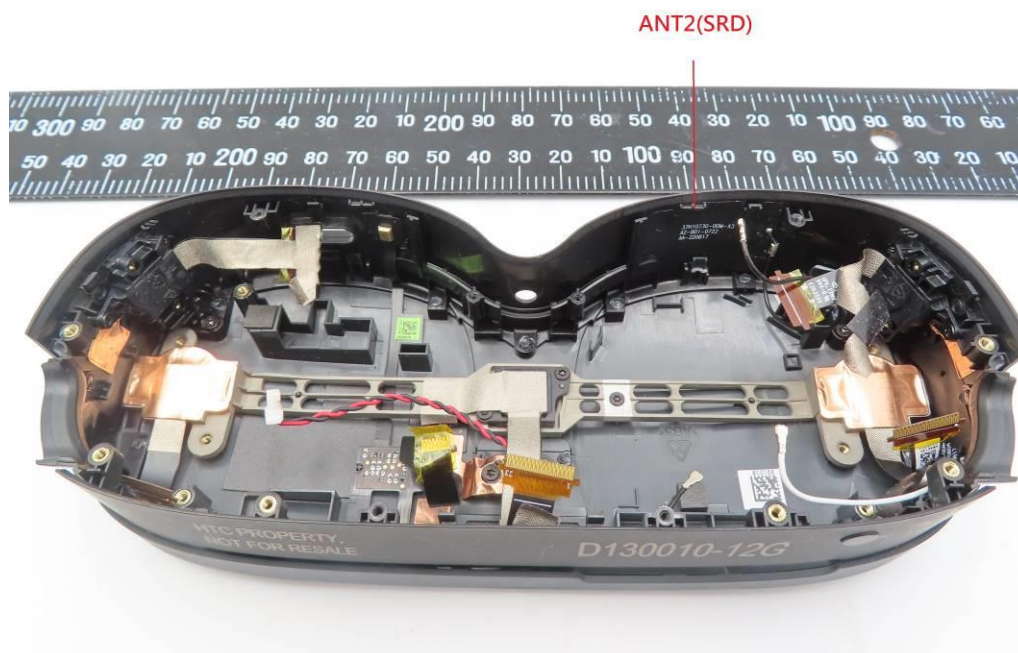
Antenna
