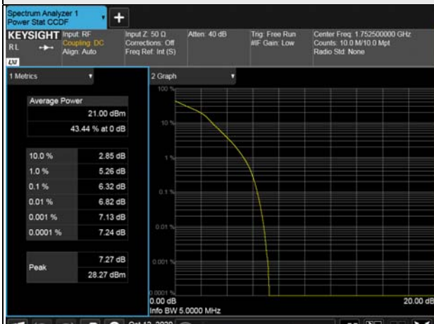
15MHz / 16QAM
