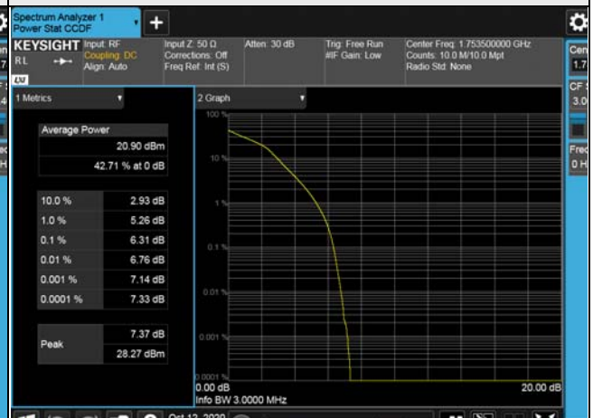
10MHz / 16QAM
