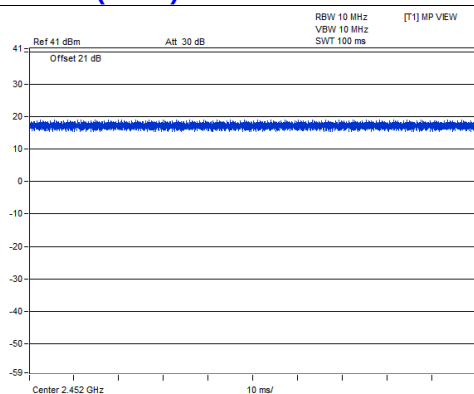
802.11n (HT40)
