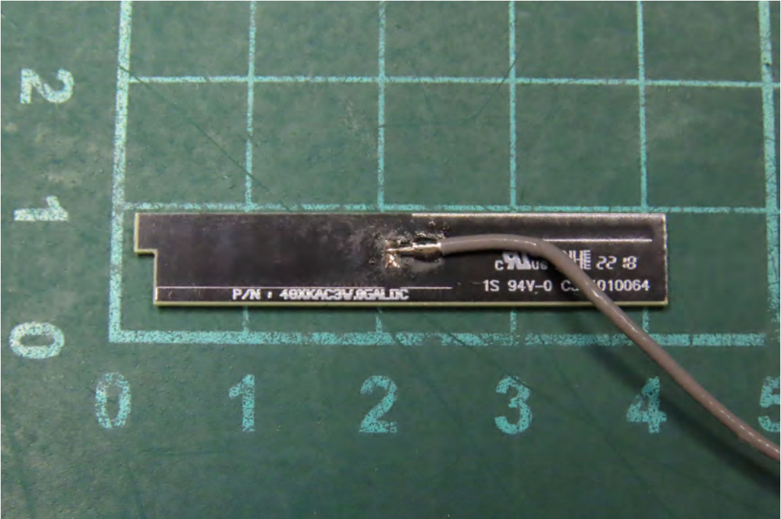
(32) EUT Photo_ BLE antenna
