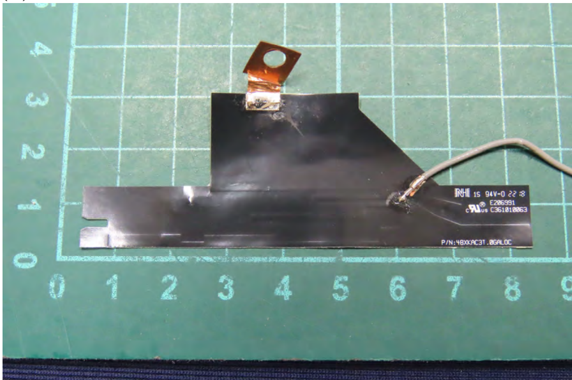
(28) EUT Photo_ LTE/FR1 Ant 1
