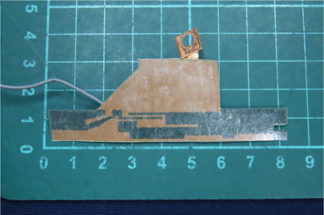
(29) EUT Photo_ LTE/FR1 Ant 1
