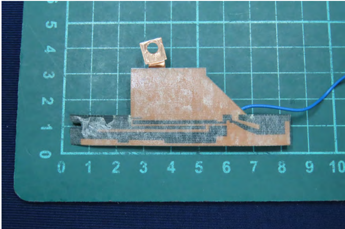
(27) EUT Photo_ LTE/FR1 Ant 3
