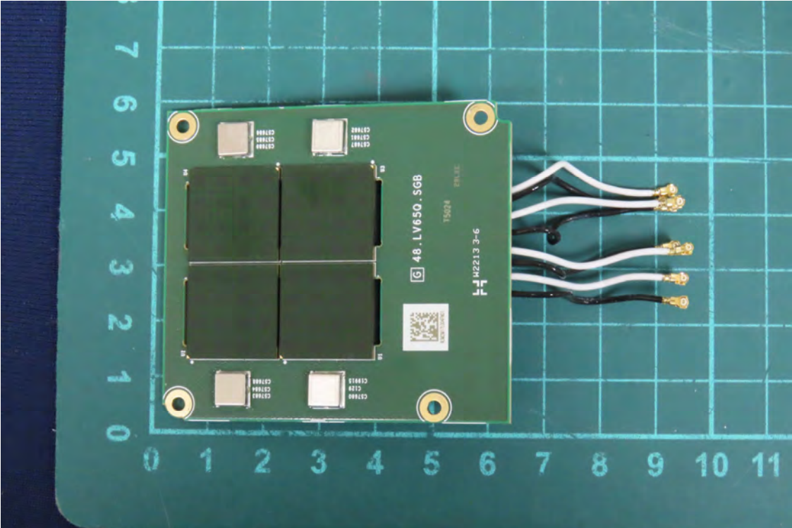
(9) EUT Photo_5G FR2 Array antenna
