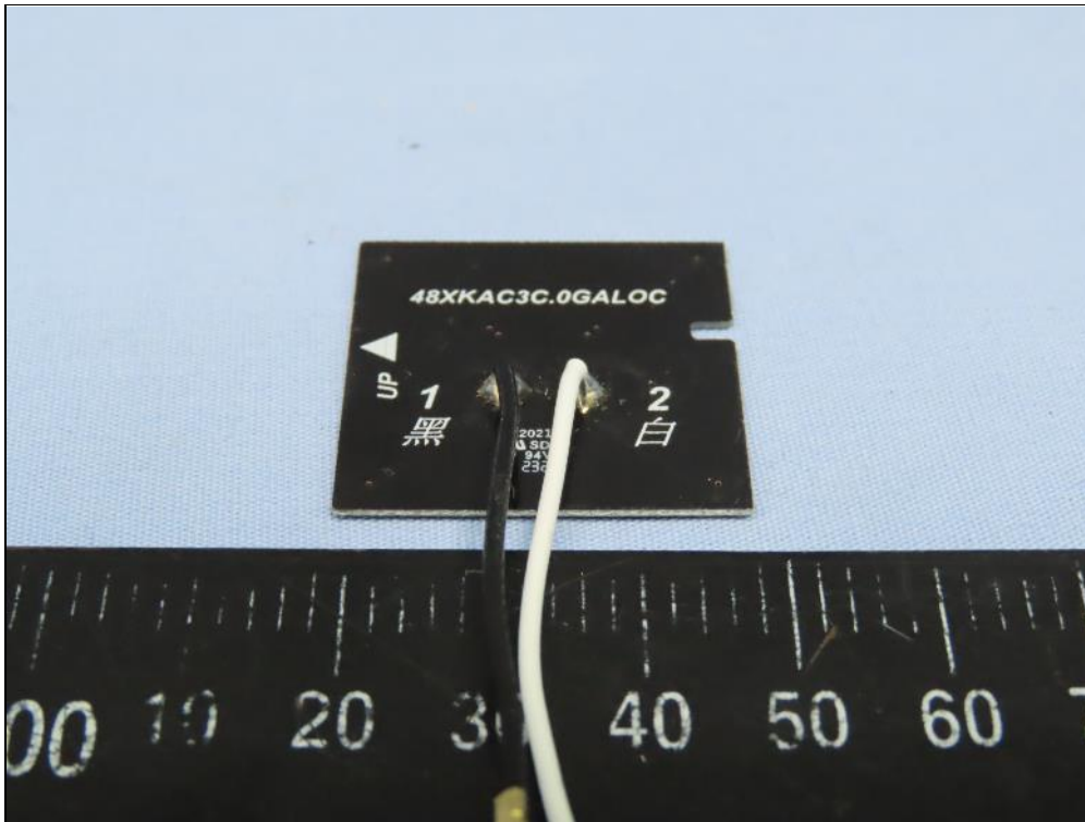
WIFI1 ANT
