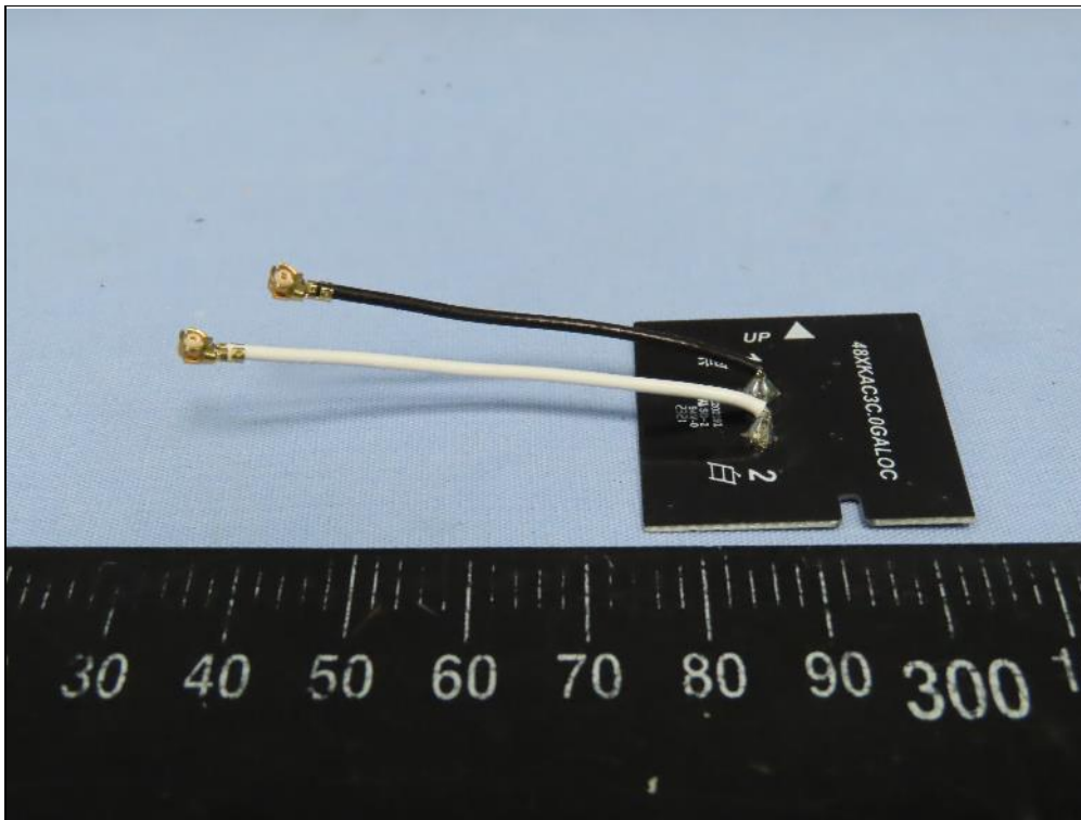
WIFI2 ANT
