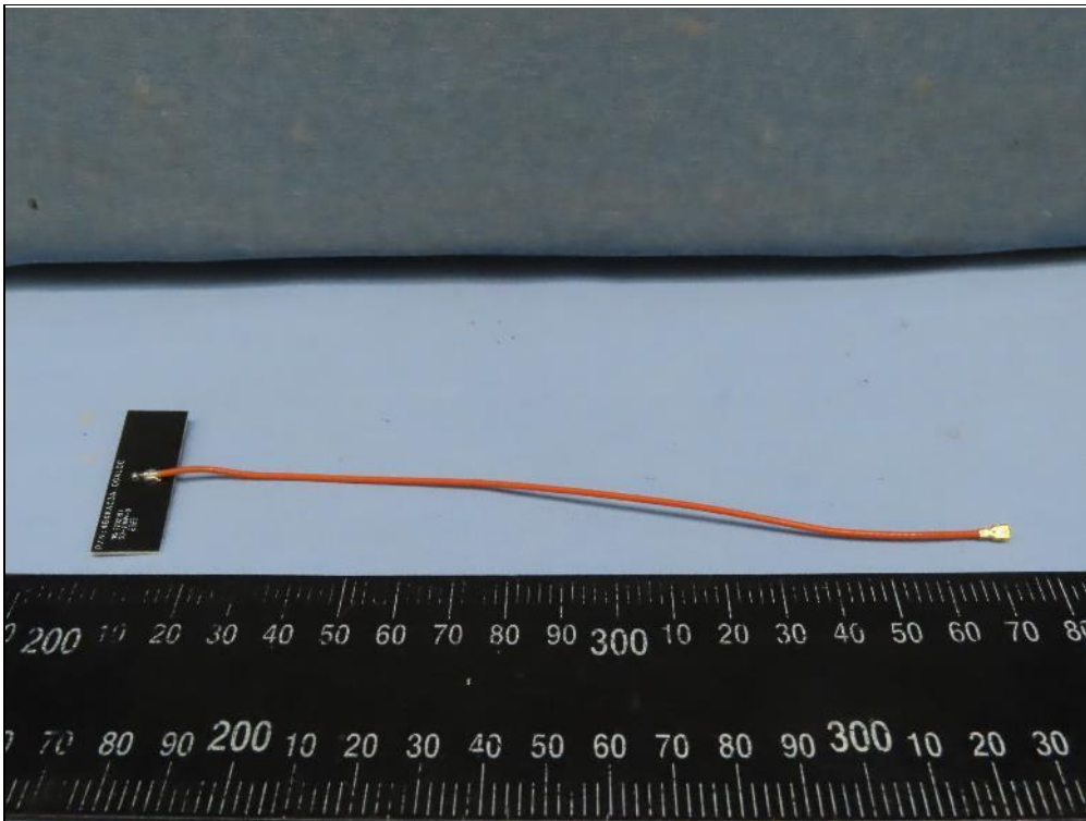
DECT2 ANT
