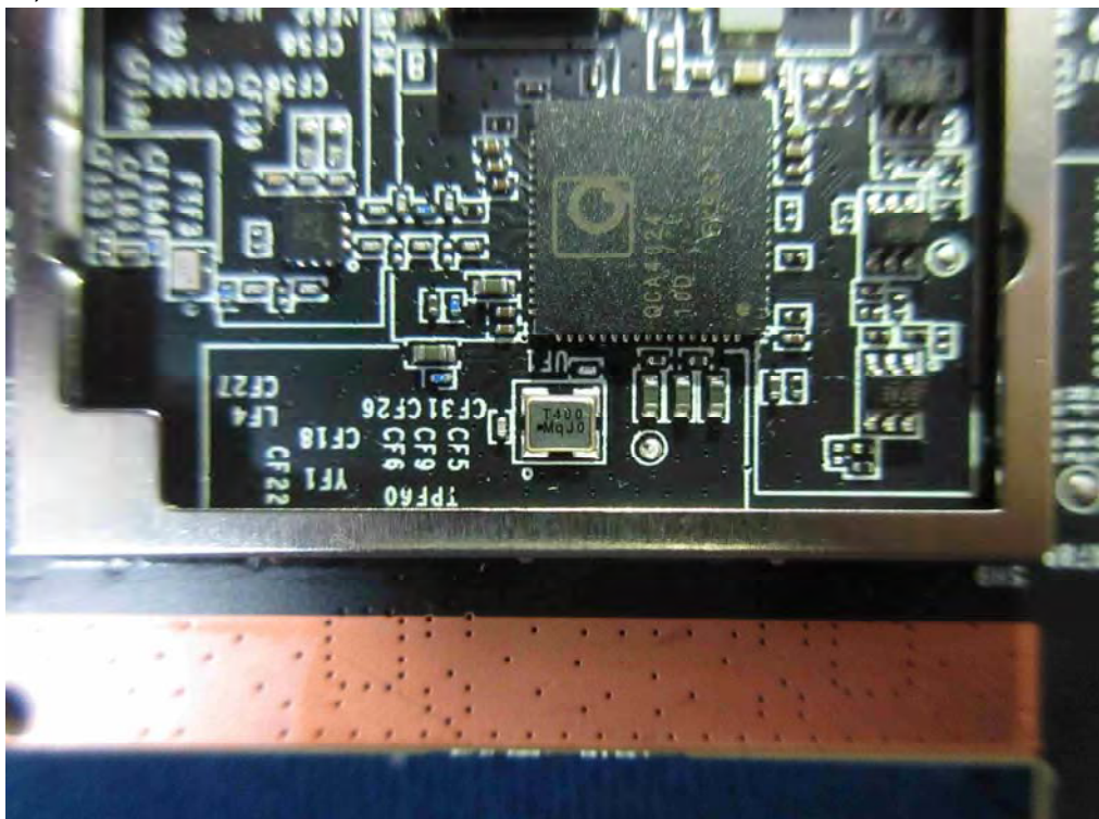
(108) EUT Photo
