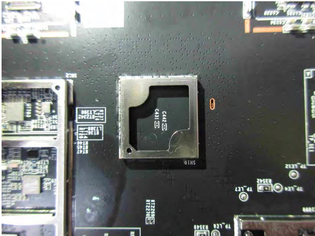
(120) EUT Photo
