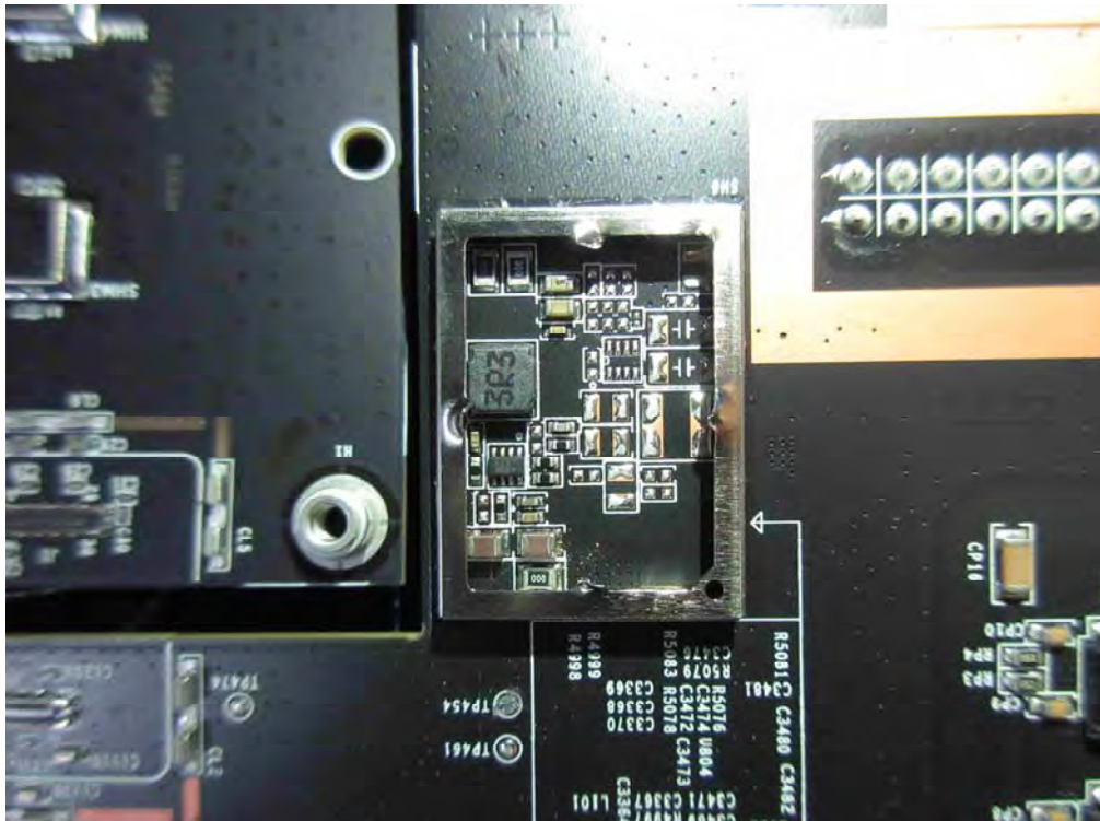
(124) EUT Photo
