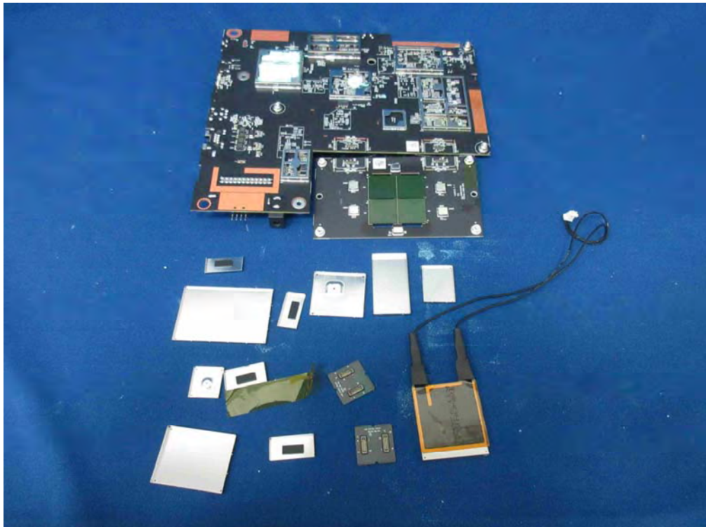
(104) EUT Photo
