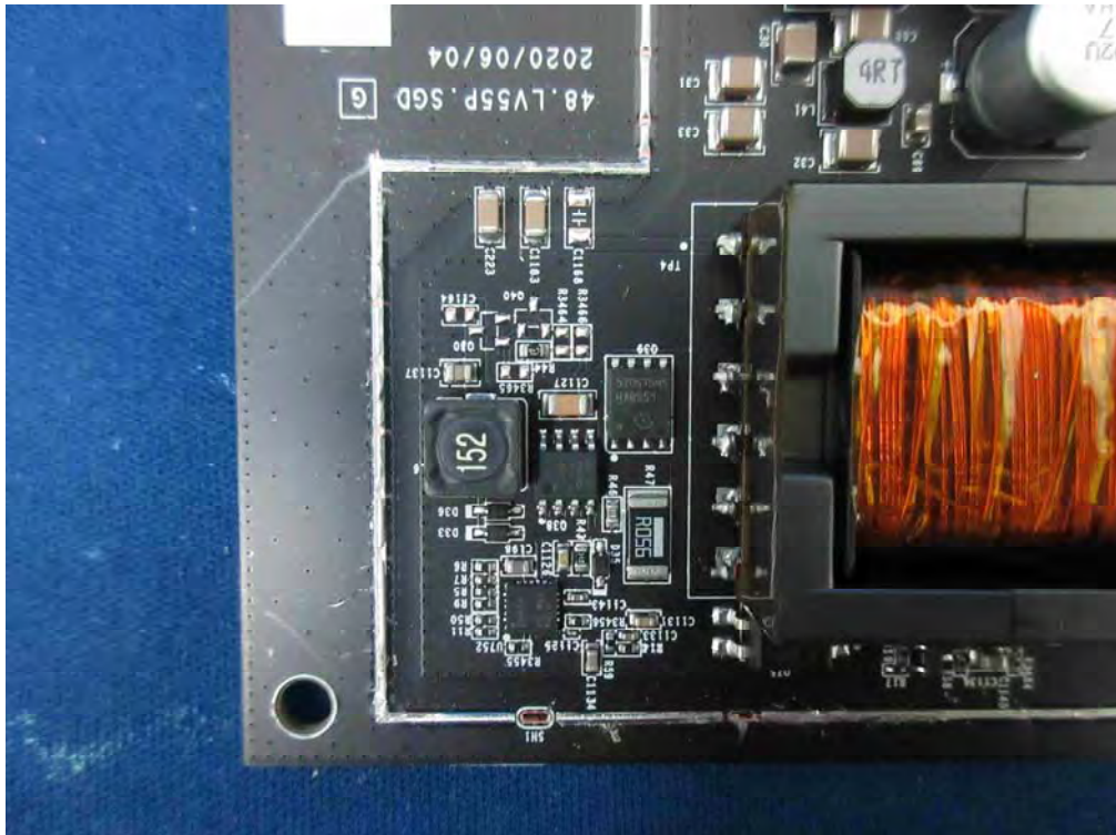
(146) EUT Photo
