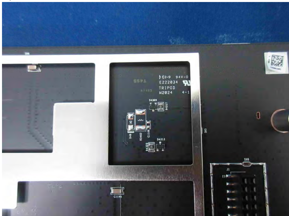
(140) EUT Photo
