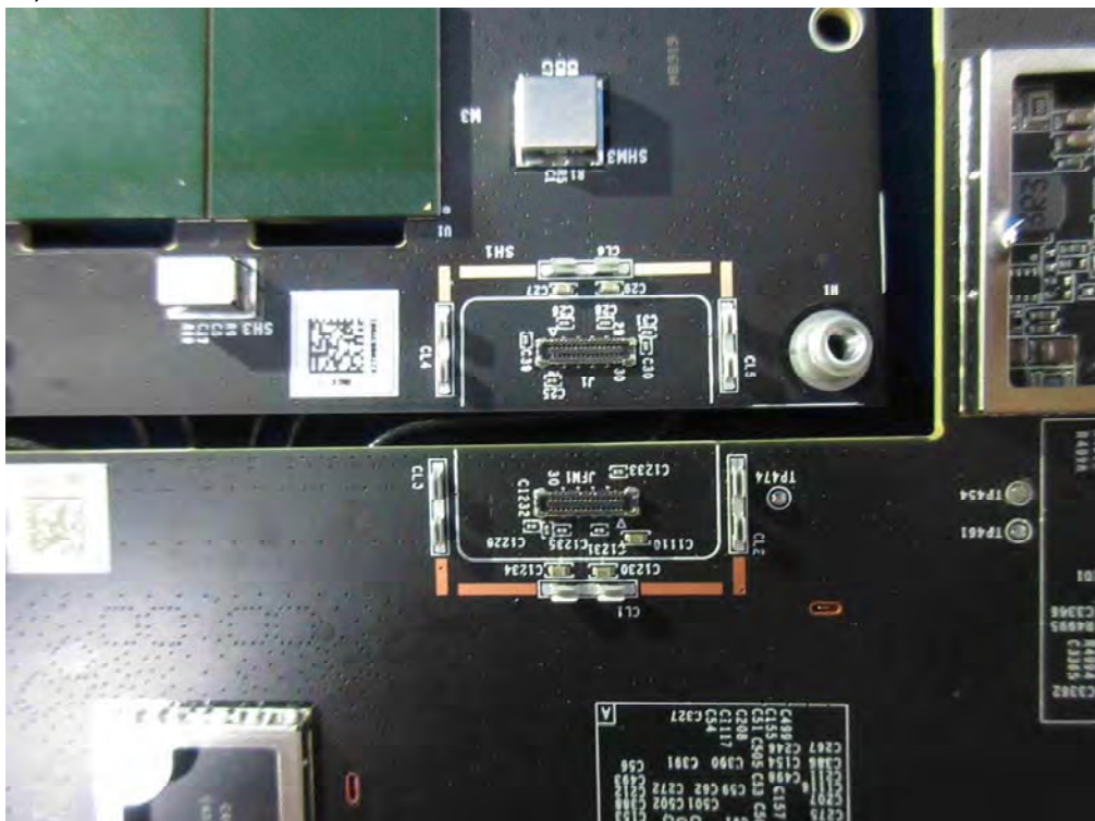
(118) EUT Photo
