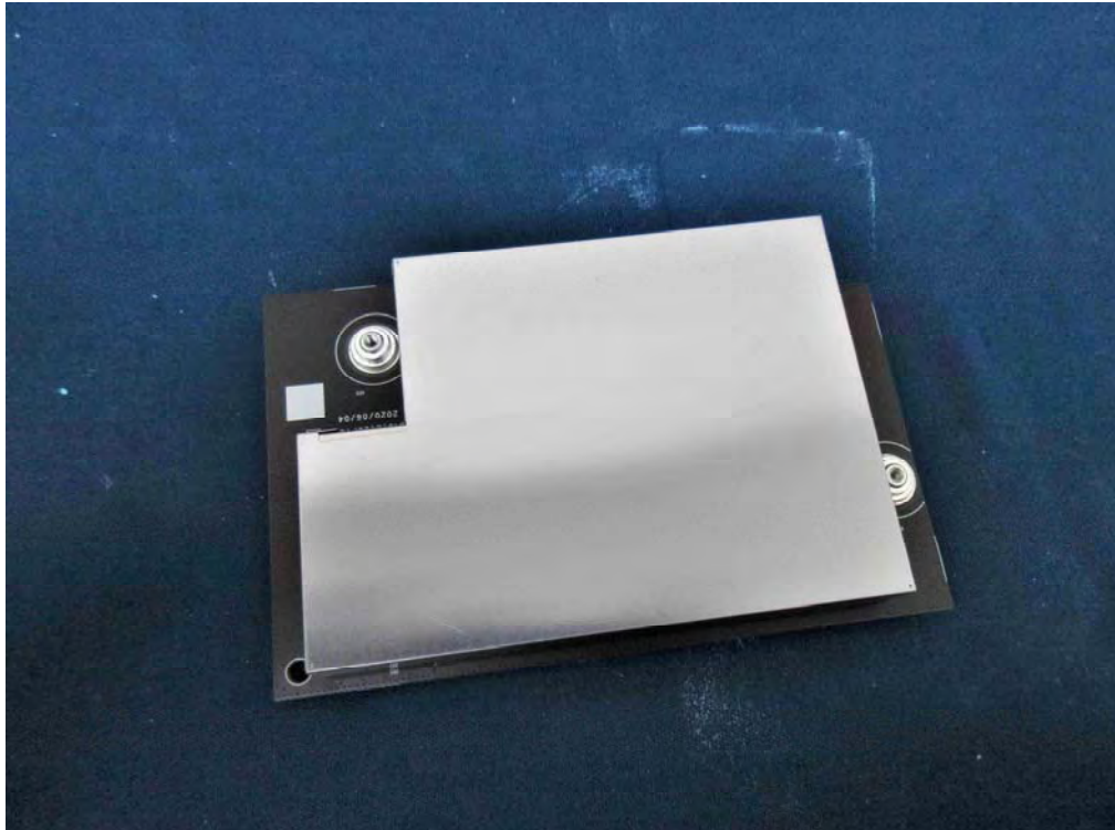
(134) EUT Photo
