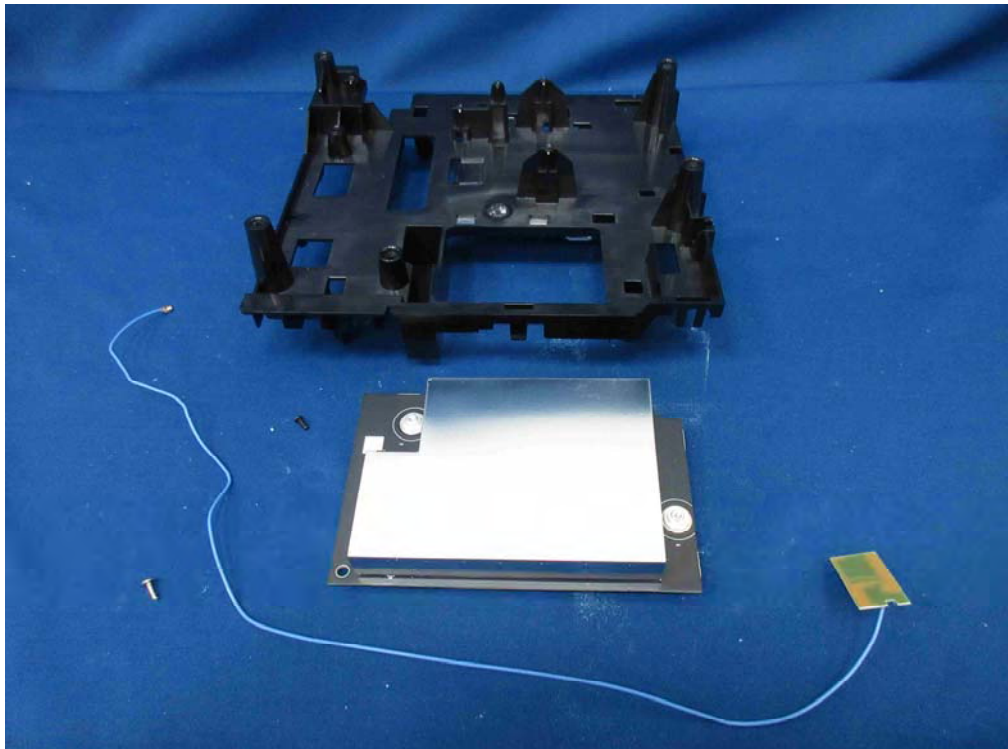
(128) EUT Photo
