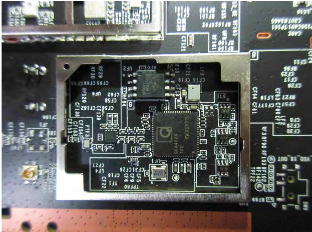
(108) EUT Photo
