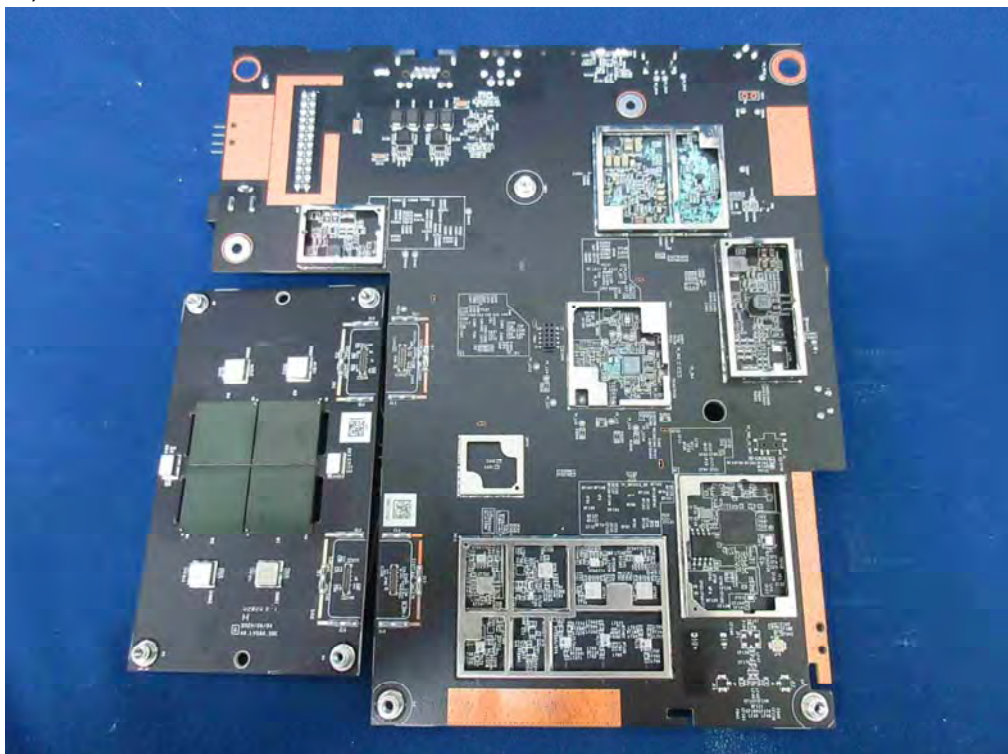
(106) EUT Photo
