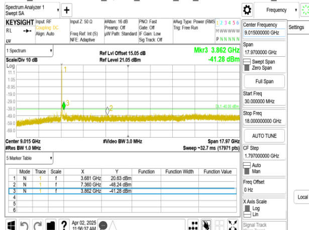
Band48_20MHz+20MHz_QPSK_RB1-99_1-0_CH56442-56640_upper 18G
