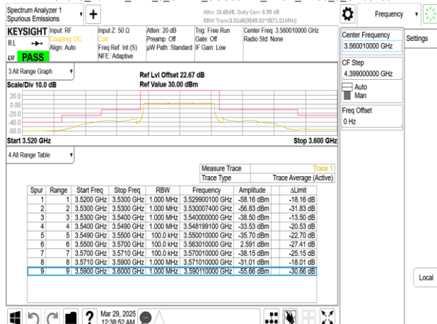
Band48_20MHz_DFT_s_OFDM_SCS30kHz_BPSK_RB1_0_CH641668
