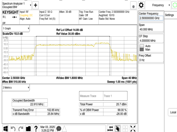
Band41_10MHz+20MHz_QPSK_RB50-0+RB100-0_CH40526+CH40670
