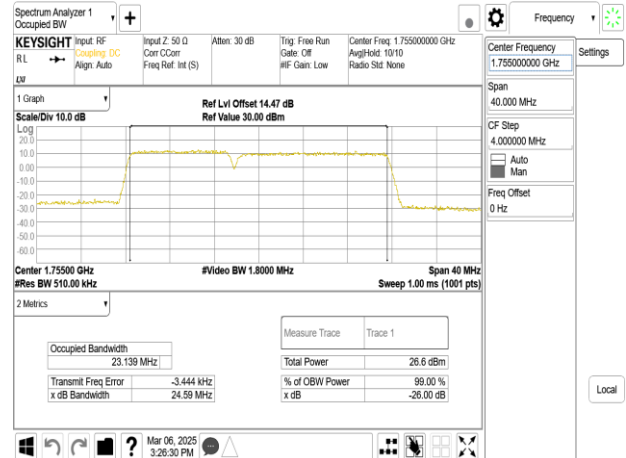
Band66_15MHz+10MHz_QPSK_RB75-0+RB50-0_CH132373+CH132493
