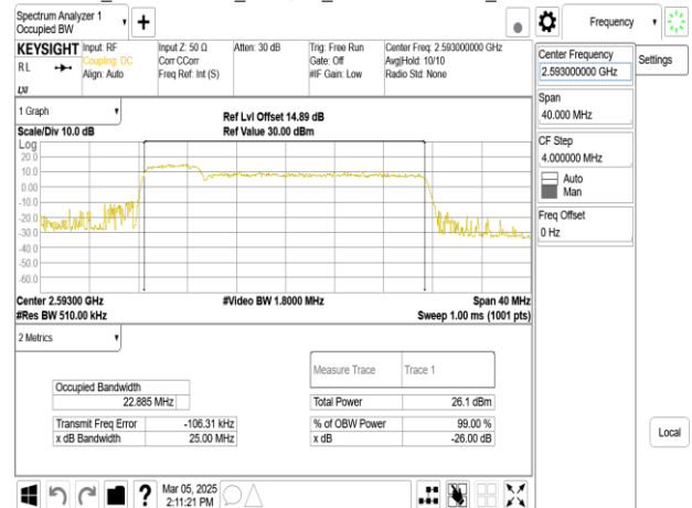
Band41_20MHz+5MHz_QPSK_RB100-0+RB25-0_CH40595+CH40712
