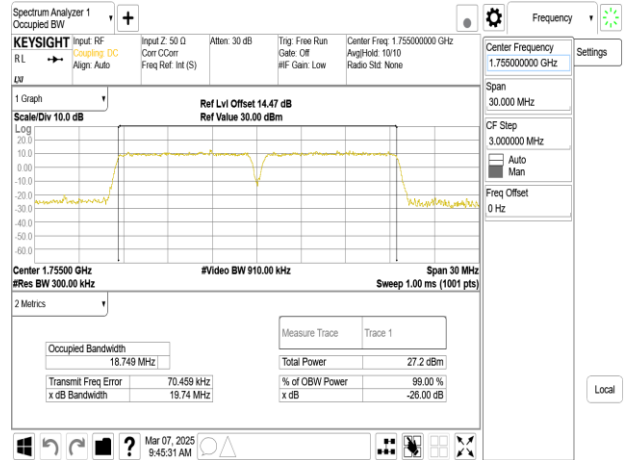
Band66B_15MHz+5MHz_QPSK_RB75-0+RB25-0_CH132398+CH132491
