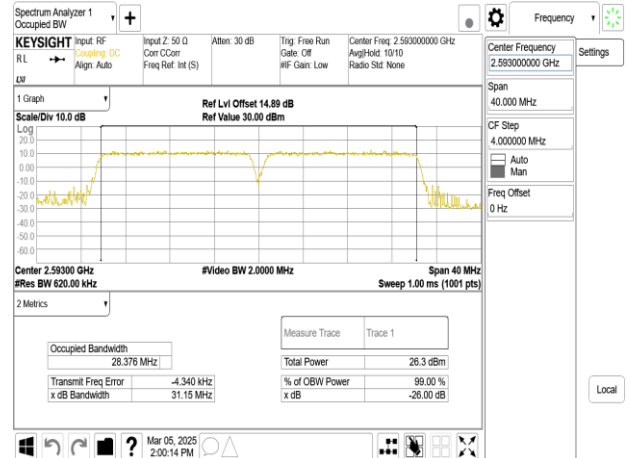
Band41_20MHz+10MHz_QPSK_RB100-0+RB50-0_CH40571+CH40715
