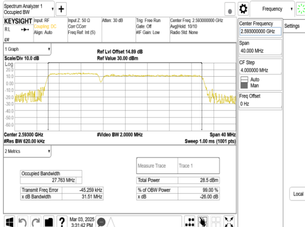
Band41_10MHz+20MHz_QPSK_RB50-0+RB100-0_CH40526+CH40670
