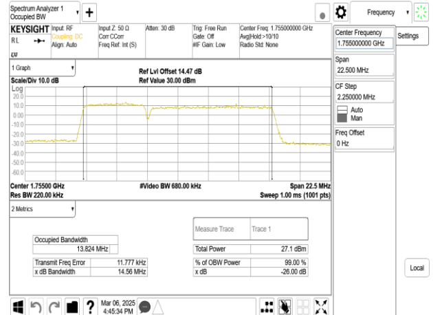
Band66B_10MHz+5MHz_QPSK_RB50-0+RB25-0_CH132397+CH132469
