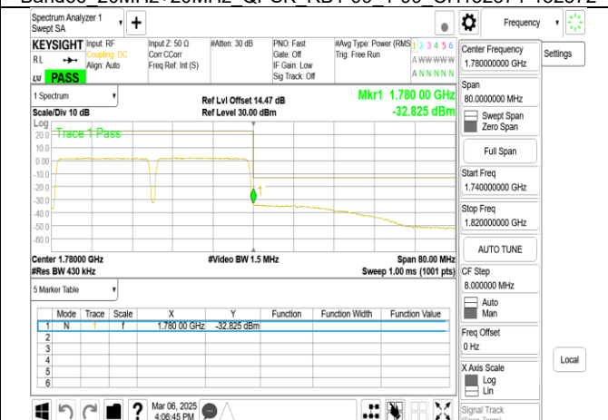
Band66_20MHz+20MHz_QPSK_RB100-0_100-0_CH132374-132572
