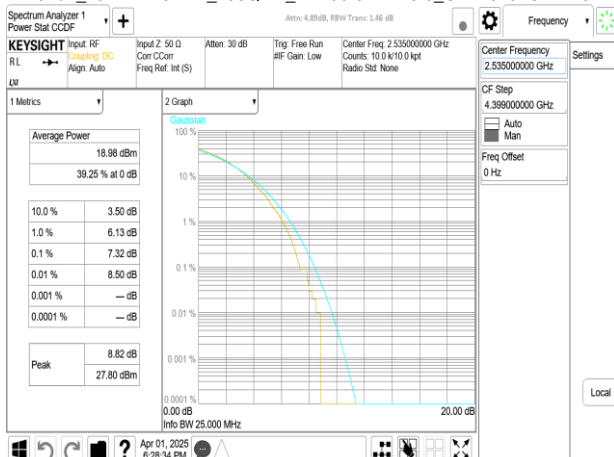
Band7_20MHz+15MHz_256QAM_RB100-0+RB75-0_CH21026+CH21197
