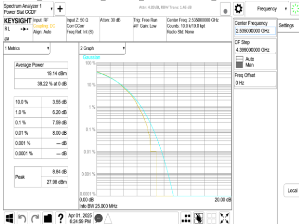
Band7_20MHz+15MHz_256QAM_RB100-0+RB75-0_CH21026+CH21197
