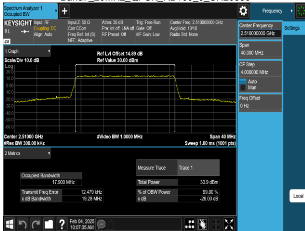
Band7_20MHz_16QAM_RB100_0_CH20850
