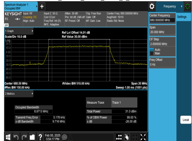
Band71_10MHz_QPSK_RB50_0_CH133297
