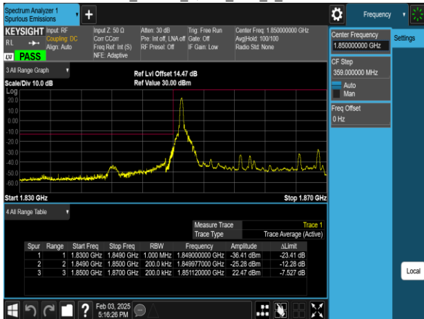
Band2_20MHz_QPSK_RB1_0_CH18700
