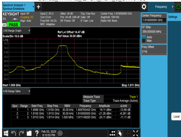
Band2_1.4MHz_QPSK_RB1_5_CH19193
