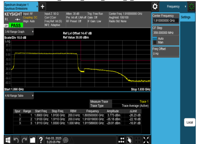
Band2_20MHz_QPSK_RB100_0_CH19100
