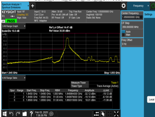
Band2_5MHz_QPSK_RB1_0_CH18625
