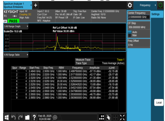
Band7 20MHz QPSK RB1_99 CH21100
