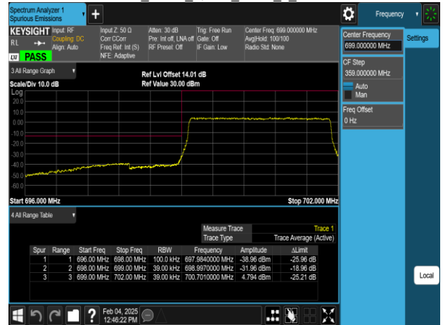
Band12_3MHz_QPSK_RB1_14_CH23165
