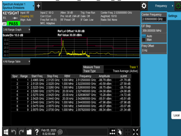
Band7_15MHz_QPSK_RB1_74_CH21100
