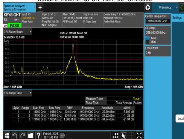
Band25_20MHz_QPSK_RB100_0_CH26590
