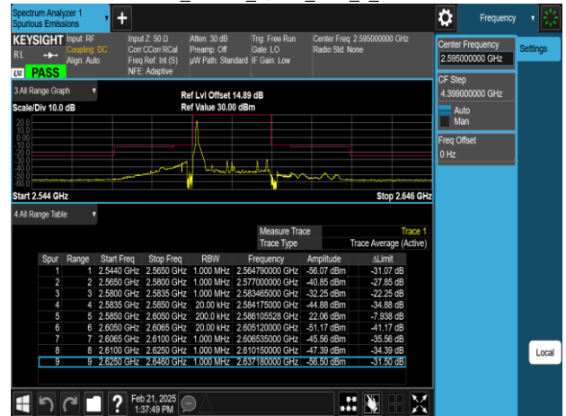
Band38_20MHz_QPSK_RB1_99_CH38000
