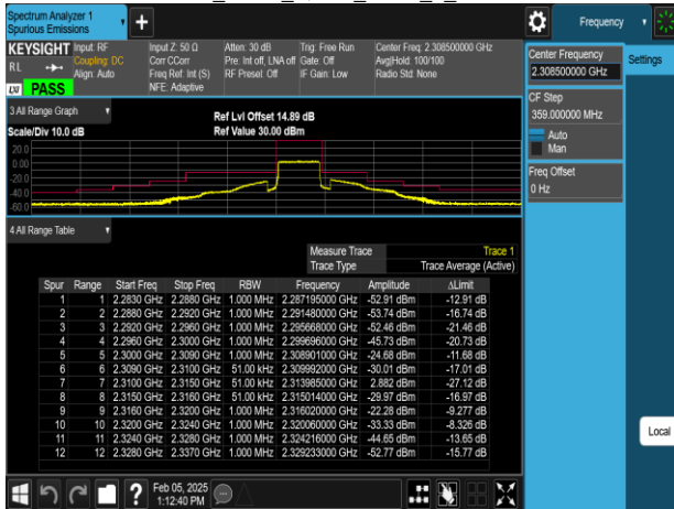
Band30_10MHz_QPSK_RB1_0_CH27710
