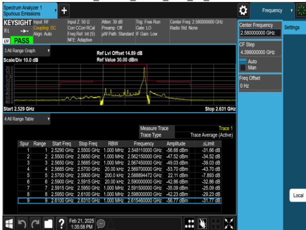
Band38_20MHz_QPSK_RB1_99_CH37850
