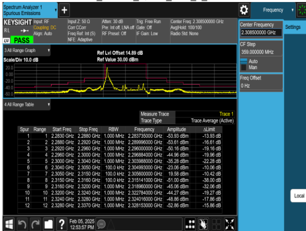
Band30_10MHz_QPSK_RB1_49_CH27710
