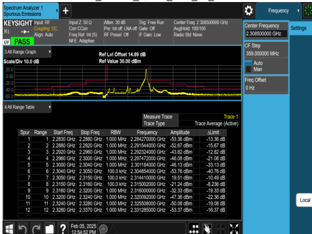
Band30_10MHz_QPSK_RB1_49_CH27710
